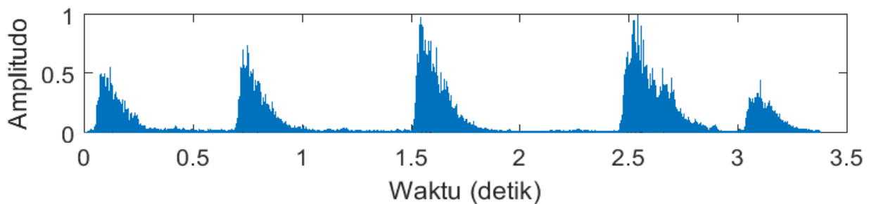
Gambar 4.6 Normalisasi
