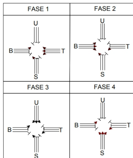
Gambar 5. 26 Pengaturan Fase Lalu Lintas Alternatif 2 Jam Lembang Simpang Gondomanan
