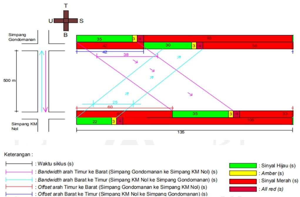
Gambar 5. 28 Diagram Sinyal Alternatif 2 Setelah Dikoordinasi Periode Jam Lengah
