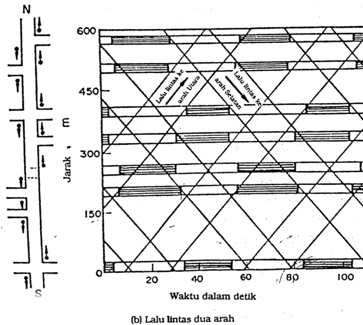
Gambar 3. 4 Koordinasi Sinyal Lampu Lalu Lintas pada Jalan Dua Arah dengan Jarak Persimpangan Tidak Seragam (Sumber: Hoobs, 1995)
