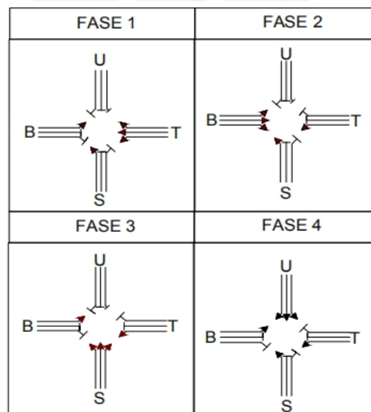
Gambar 5. 23 Pengaturan Fase Lalu Lintas Alternatif 1 Jam Lembang Simpang Gondomanan
