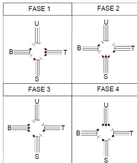
Gambar 5. 17 Pengaturan Fase Lalu Lintas Alternatif 1 Jam Puncak Simpang Gondomanan
