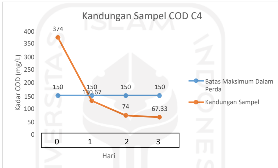
Gambar 4.10 Grafik Penurunan COD C 4 Dengan Treatment Filtrasi
