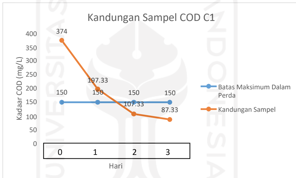
Gambar 4.1 Grafik Penurunan COD C 1 Dengan Treatment Fitoremediasi
