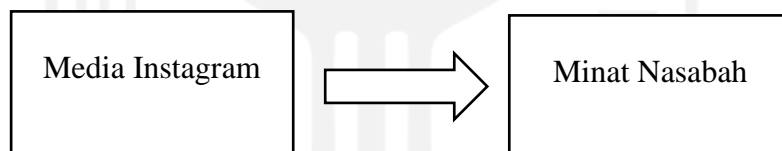
Gambar 1: Kerangka Berpikir
