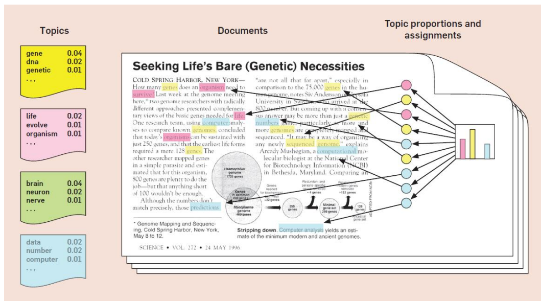
Gambar 2.3 Gambaran Konsep LDA (Blei, 2012)
