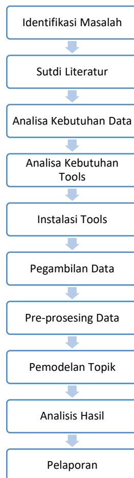
Gambar 3.1 Alur Metodologi Penelitian
