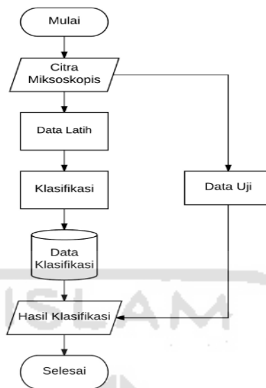
Gambar 4.4 Flowchart Klasifikasi
