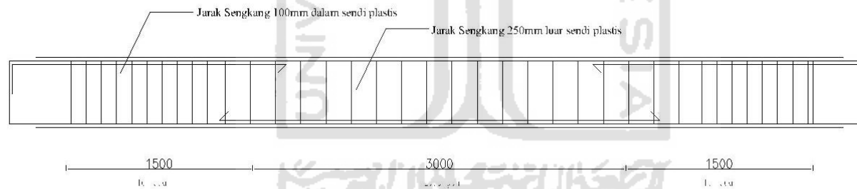
POTONGAN MEMANJANG Ba1 LANTAI 1
