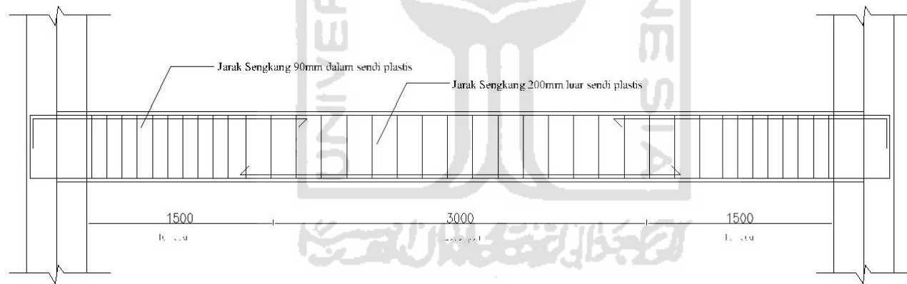
POTONGAN MEMANJANG B1 LANTAI 3
