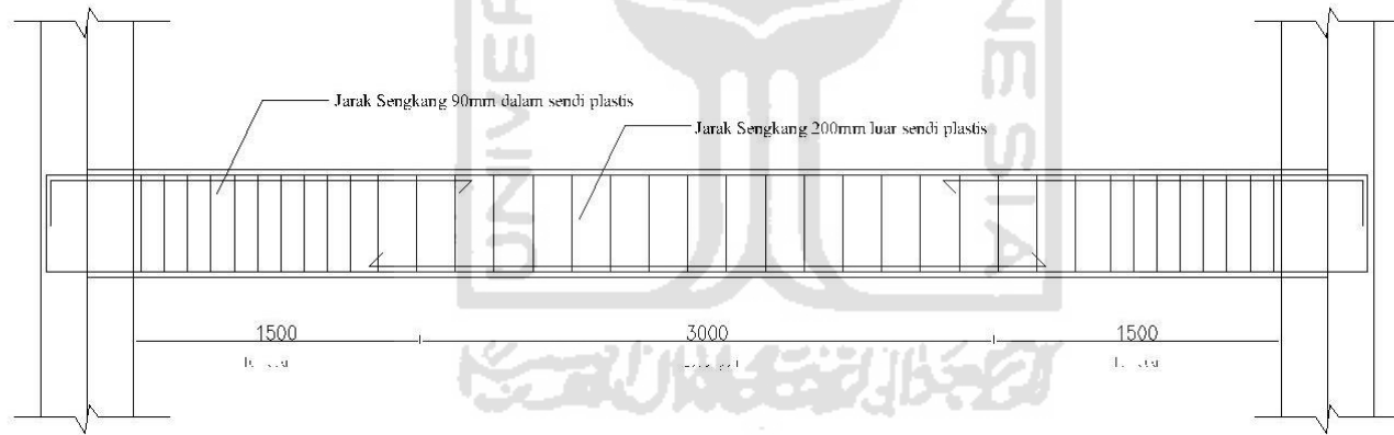
POTONGAN MEMANJANG B1 LANTAI 4
