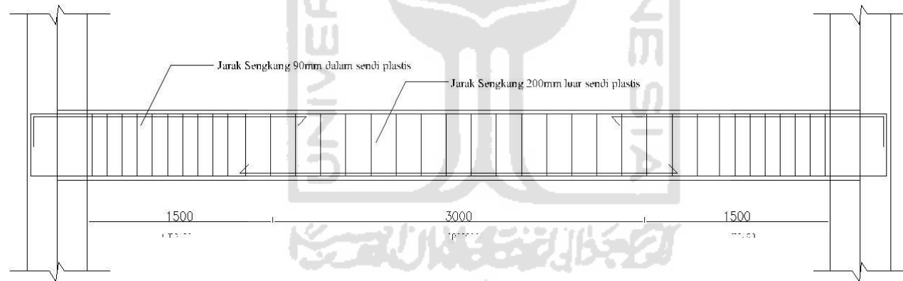
POTONGAN MEMANJANG B1 LANTAI 1
