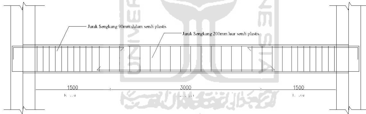
POTONGAN MEMANJANG B1 LANTAI 2
