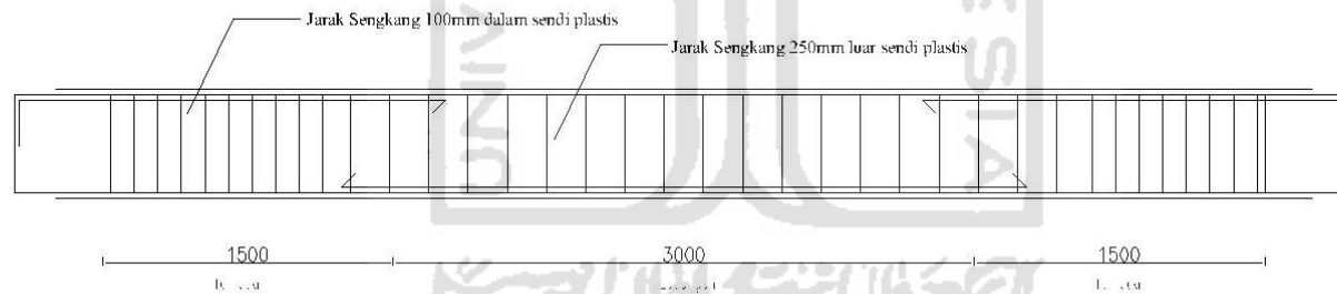
POTONGAN MEMANJANG Ba1 LANTAI 3
