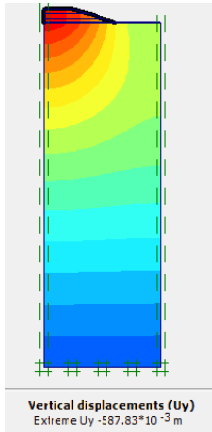
Gambar L-9.9 Jaringan Elemen Terdeformasi Vertikal Timbunan 3 m, Tanah Asli 70 m
