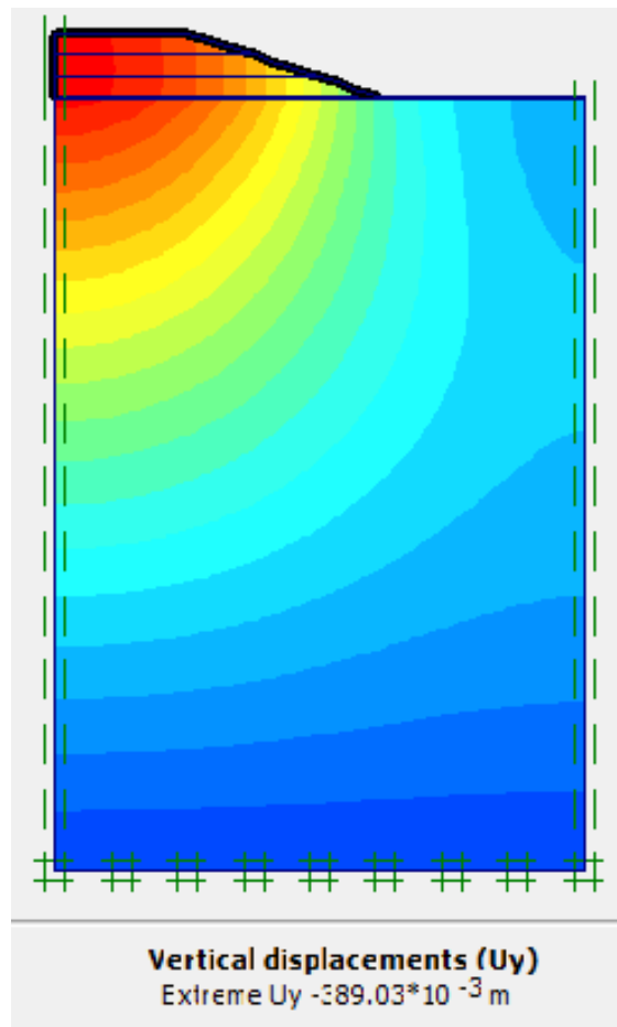
Gambar L-9.8 Jaringan Elemen Terdeformasi Vertikal Timbunan 3 m, Tanah Asli 35 m
