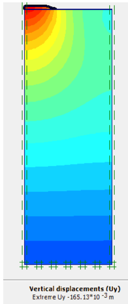
Gambar L-9.3 Jaring Elemen Terdeformasi Vertikal Timbunan 1 m, Tanah Asli 70 m
