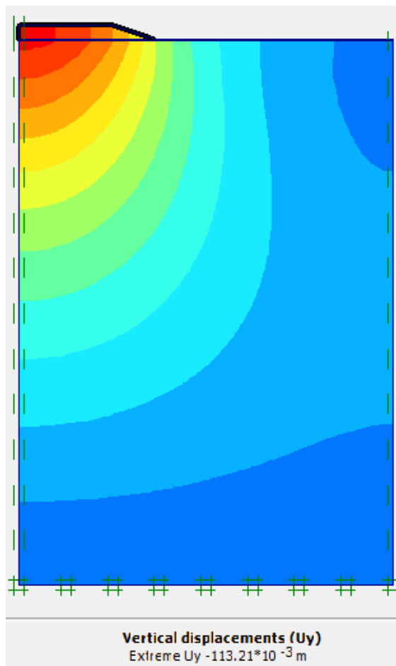
Gambar L-9.2 Jaringan Elemen Terdeformasi Vertikal Timbunan 1 m, Tanah Asli 35 m
