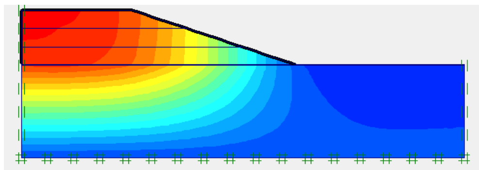
Gambar L-9.7 Jaringan Elemen Terdeformasi Vertikal Timbunan 3 m, Tanah Asli 5 m
