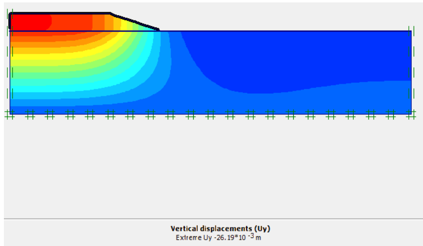
Gambar L-9.1 Jaringan Elemen Terdeformasi Vertikal Timbunan 1 m, Tanah Asli 5 m
