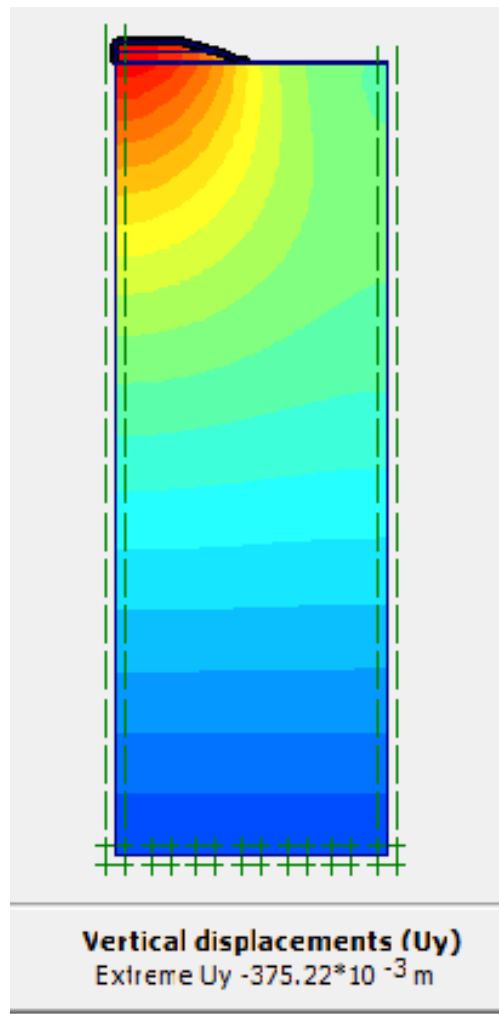
Gambar L-9.6 Jaringan Elemen Terdeformasi Vertikal Timbunan 2 m, Tanah Asli 70 m
