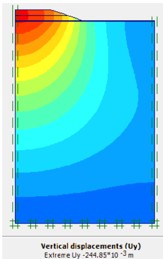
Gambar L-9.5 Jaringan Elemen Terdeformasi Vertikal Timbunan 2 m, Tanah Asli 35 m
