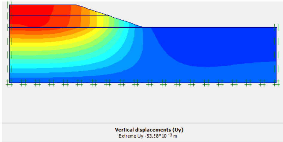
Gambar L-9.4 Jaringan Elemen Terdeformasi Vertikal Timbunan 2 m, Tanah Asli 5 m
