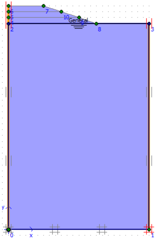
Gambar L-6.8 Kondisi Awal Timbunan 3 m, Tanah Asli 35 m
