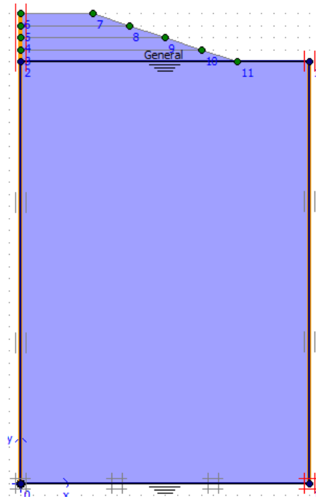
Gambar L-6.11 Kondisi Awal Timbunan 4 m, Tanah Asli 35 m
