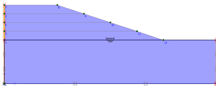
Gambar L-6.10 Kondisi Awal Timbunan 4 m, Tanah Asli 5 m
