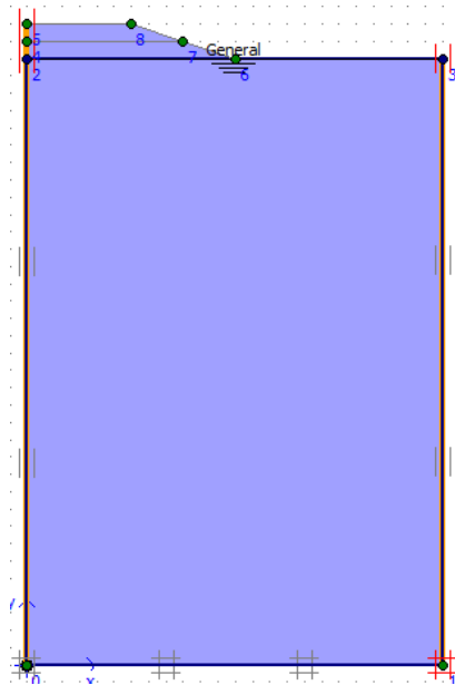
Gambar L-6.5 Kondisi Awal Timbunan 2 m, Tanah Asli 35 m
