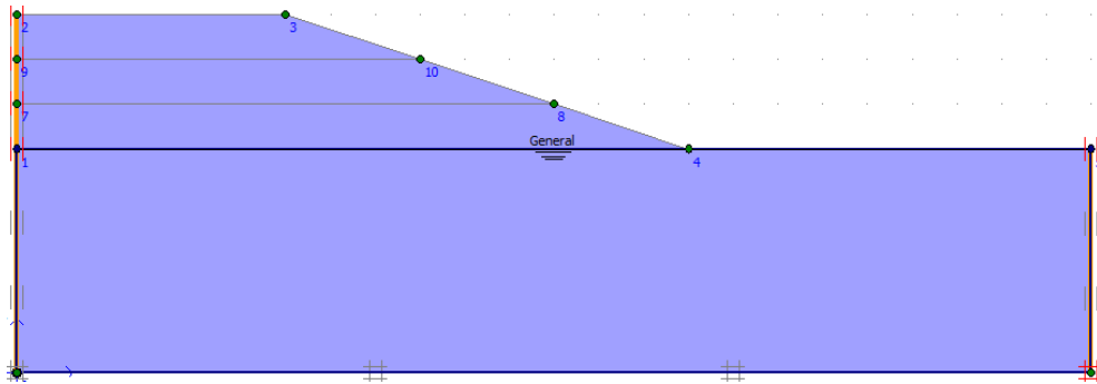
Gambar L-6.7 Kondisi Awal Timbunan 3 m, Tanah Asli 5 m
