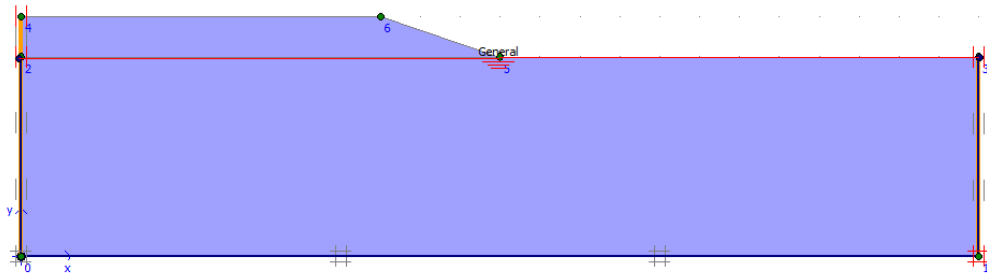
Gambar L-6.1 Kondisi Awal Timbunan 1 m, Tanah Asli 5 m
