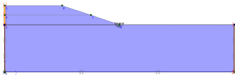
Gambar L-6.4 Kondisi Awal Timbunan 2 m, Tanah Asli 5 m
