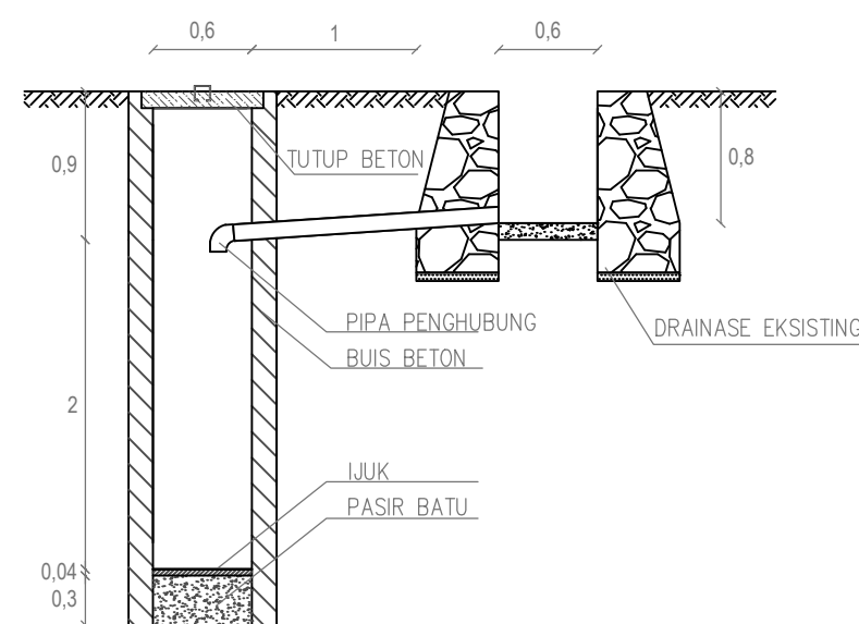
POTONGAN A-A SALURAN 25
