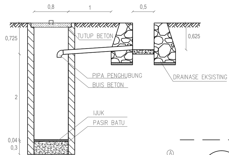
POTONGAN A-A SALURAN 16
