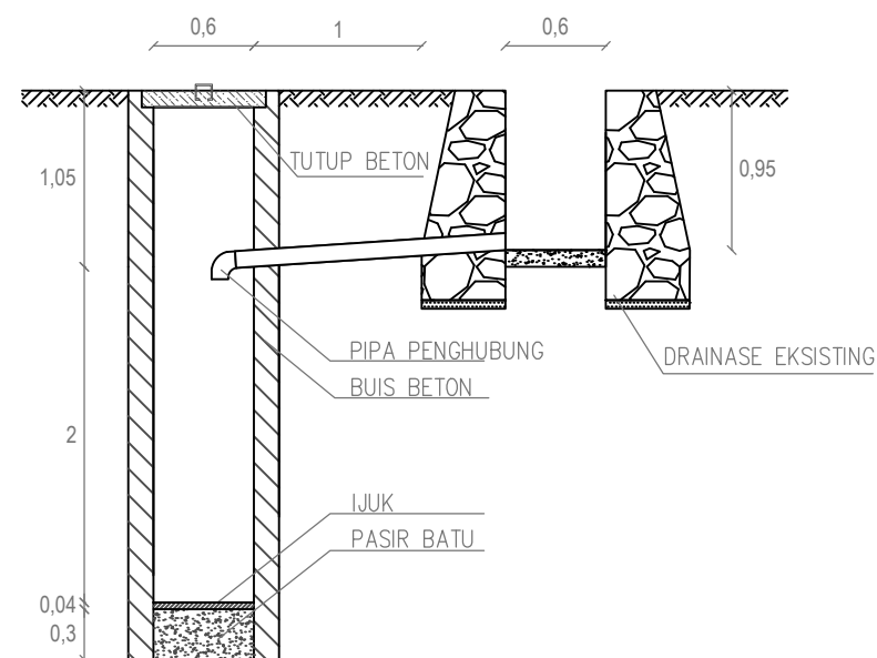
POTONGAN A-A SALURAN 18
