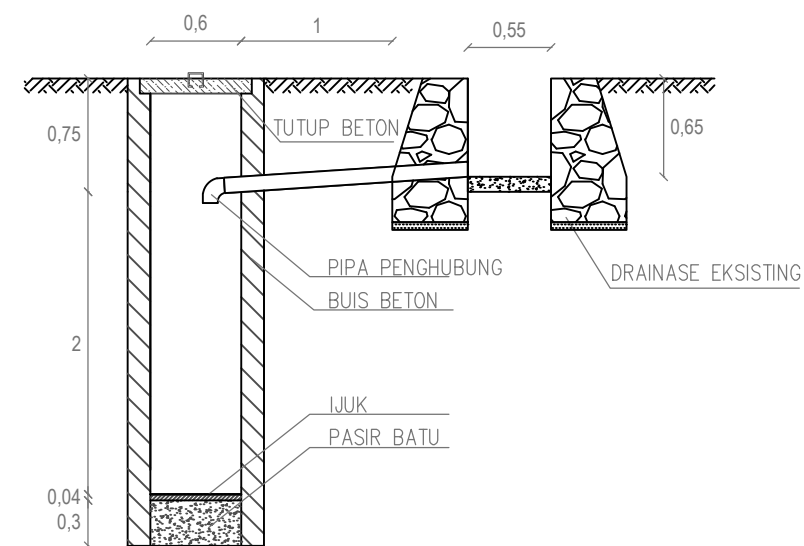
POTONGAN A-A SALURAN 14
