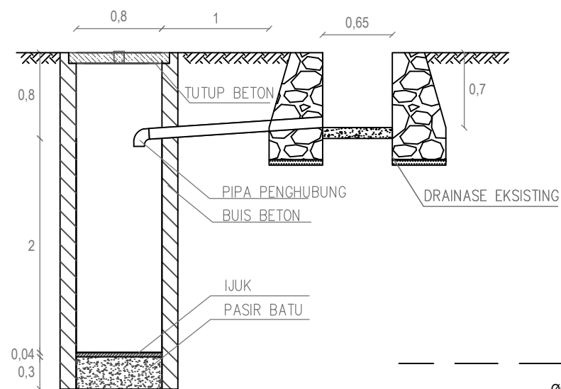
POTONGAN A-A SALURAN 13
