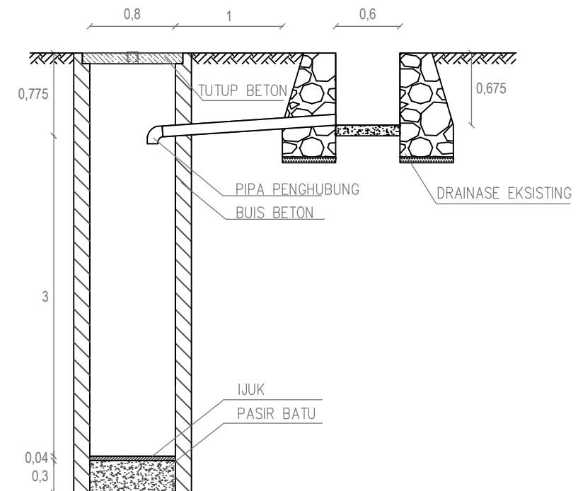
POTONGAN A-A SALURAN 11
