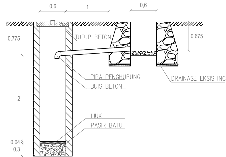
POTONGAN A-A SALURAN 12
