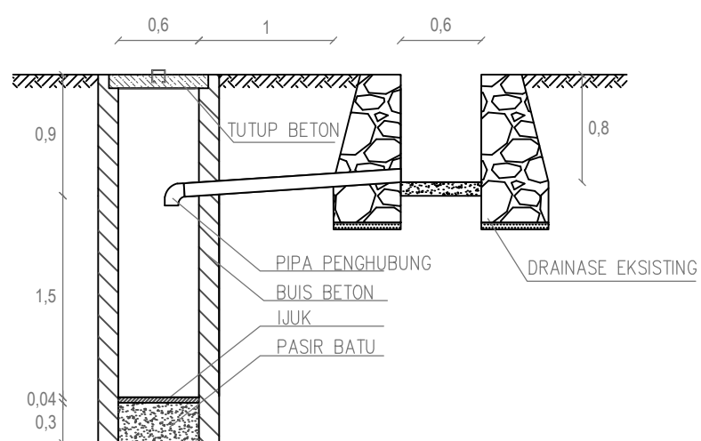
POTONGAN A-A SALURAN 24
