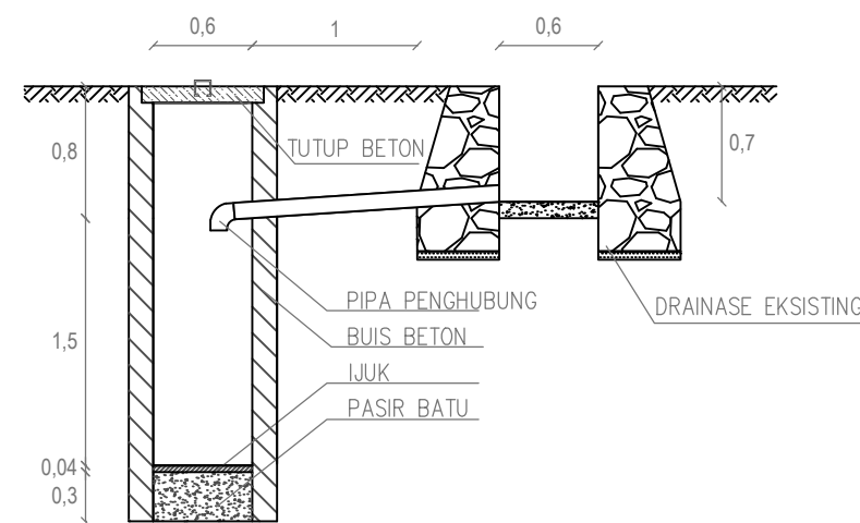
POTONGAN A-A SALURAN 5
