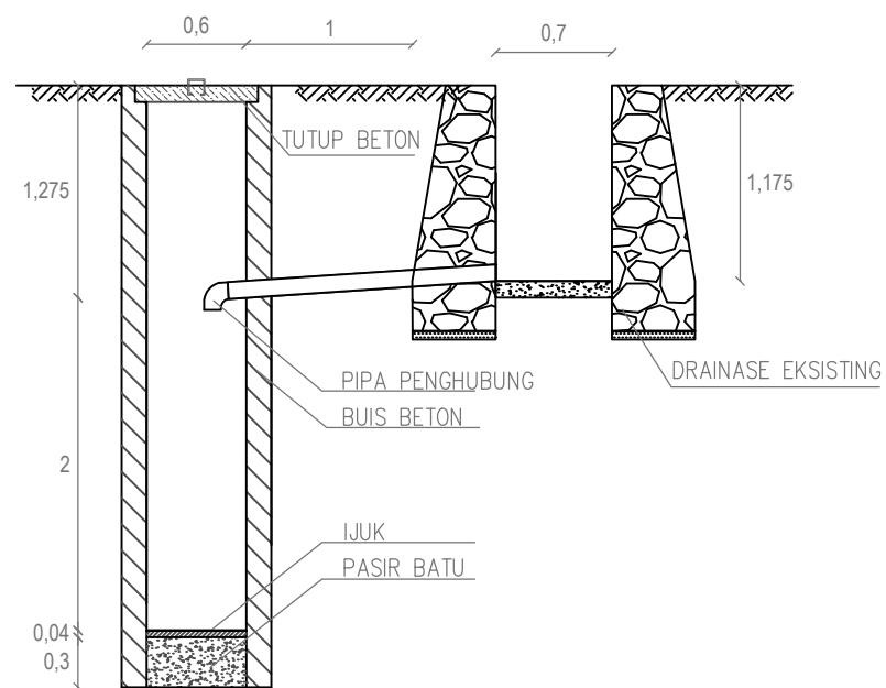
POTONGAN A-A SALURAN 15
