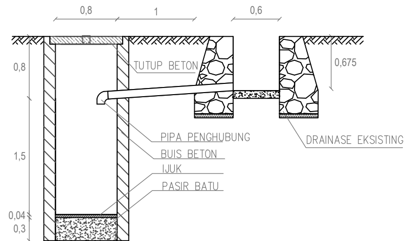
POTONGAN A-A SALURAN 10
