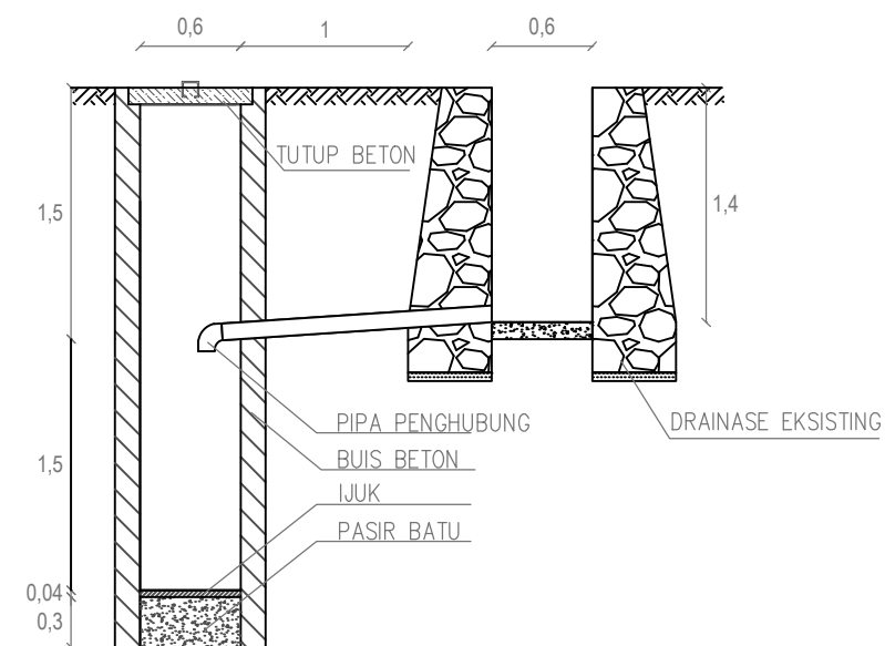
POTONGAN A-A SALURAN 8
