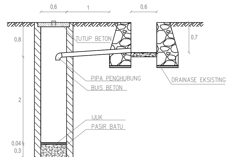
POTONGAN A-A SALURAN 2
