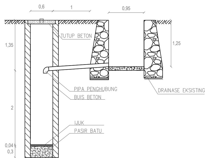
POTONGAN A-A SALURAN 3
