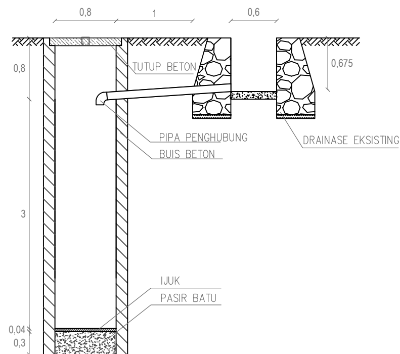
POTONGAN A-A SALURAN 9
