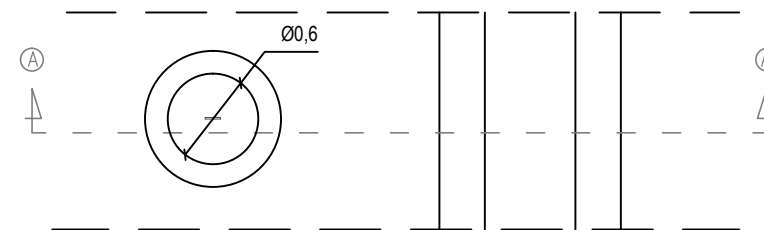
DENAH SUMUR RESAPAN SALURAN 17
