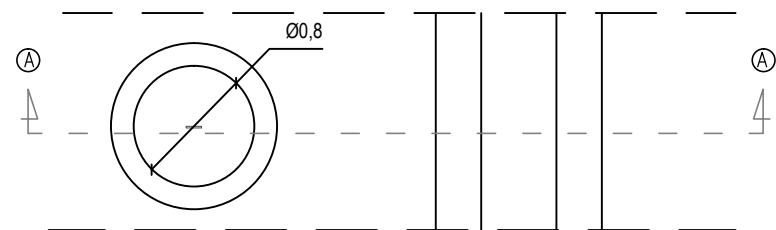
DENAH SUMUR RESAPAN SALURAN 19
