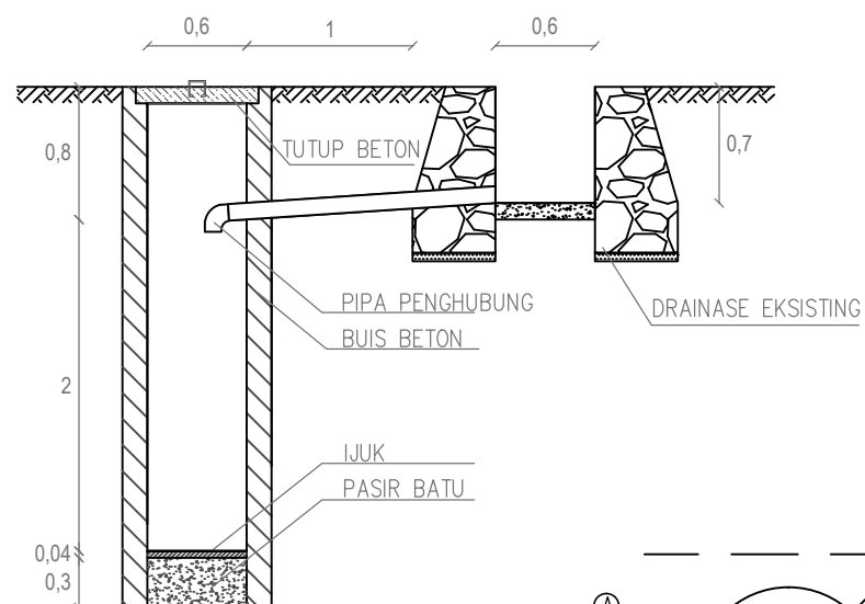
POTONGAN A-A SALURAN 4
