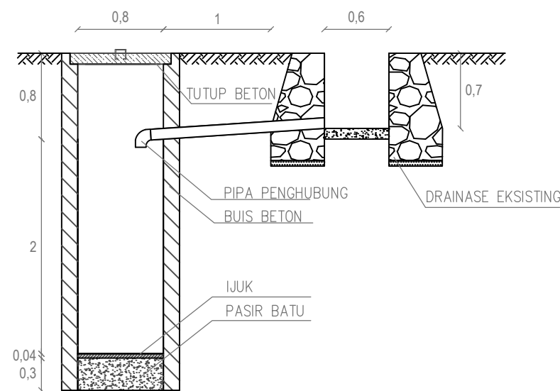
POTONGAN A-A SALURAN 6
