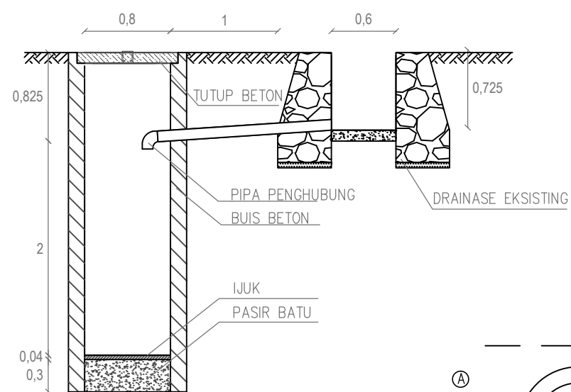
POTONGAN A-A SALURAN 7
