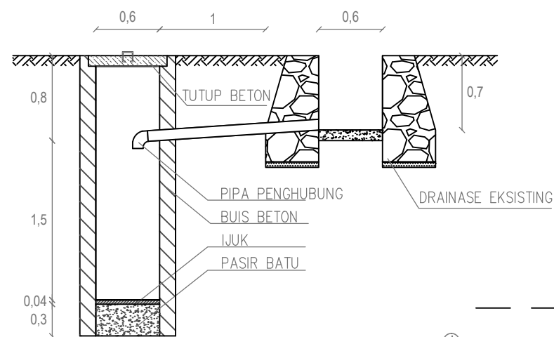
POTONGAN A-A SALURAN 1
