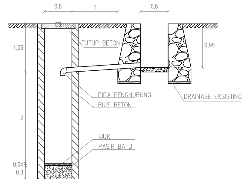
POTONGAN A-A SALURAN 17
