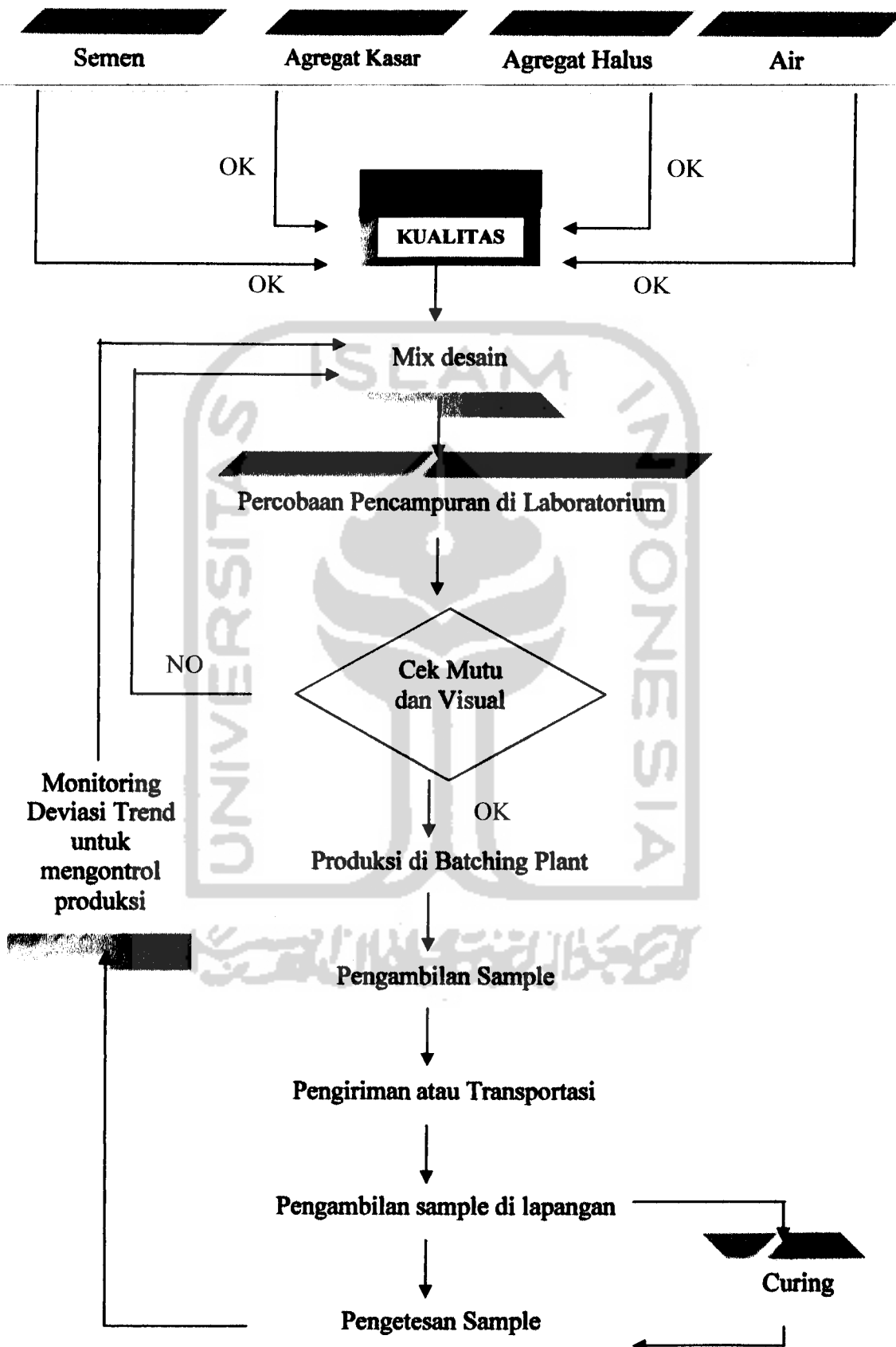
3.1 Flow Chart Produksi Beton Ready Mix
