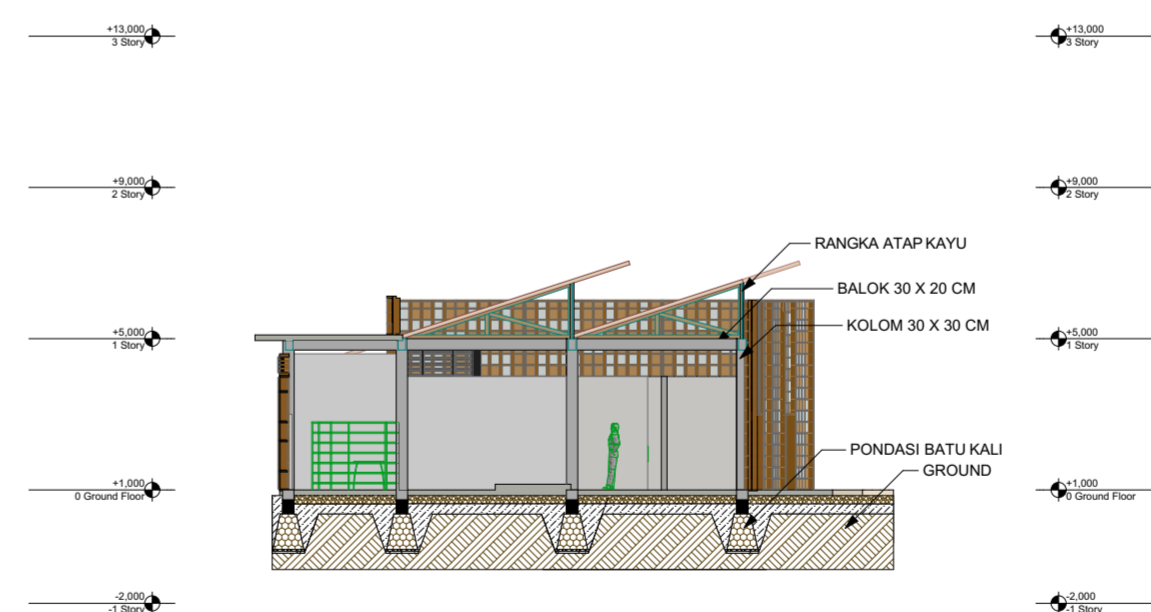
POTONGAN D SKALA 1 : 200
