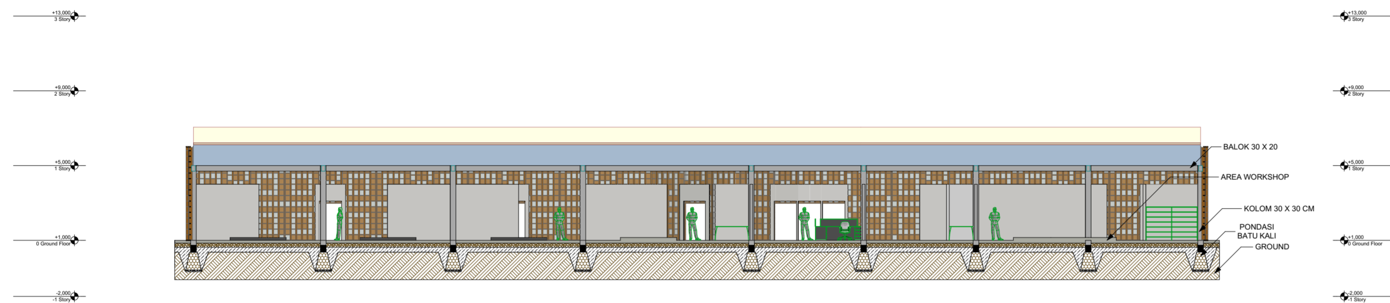
POTONGAN C SKALA 1 : 200
