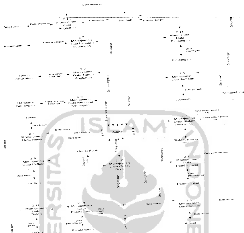
Gambar 3.4 DFD Level 2 proses manajemen data
