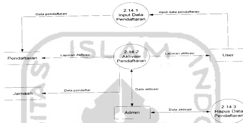
Gambar 3. 19 DFD Level 3 proses manajemen data pendaftaran
