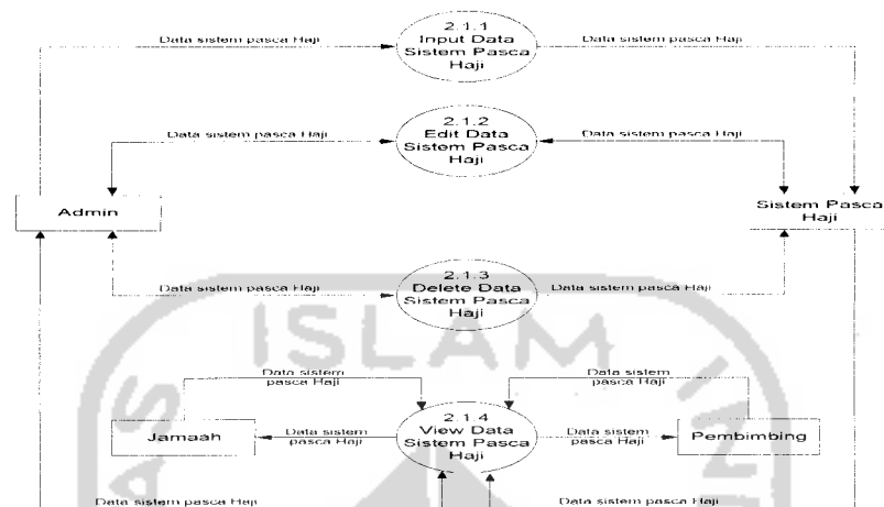
Gambar 3.6 DFD Level 3 proses manajemen data sistem pasca haji
