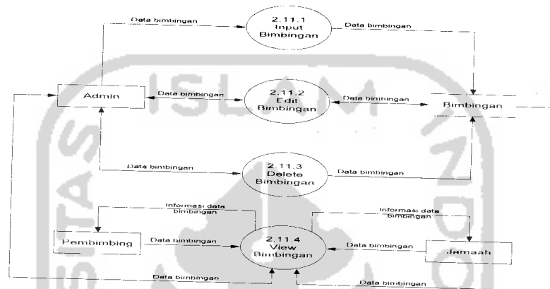
Gambar 3.16 DFD Level 3 proses manajemen data bimbingan
