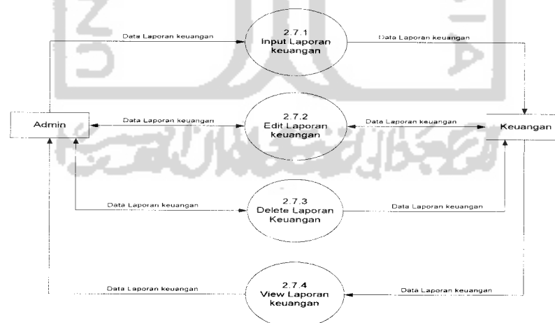
Gambar 3.12 DFD Level 3 proses manajemen data laporan keuangan
