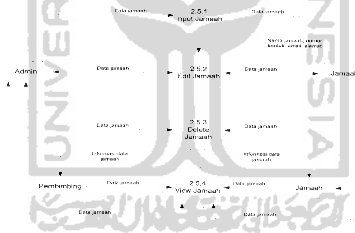
Gambar 3.10 DFD Level 3 proses manajemen data jamaah
