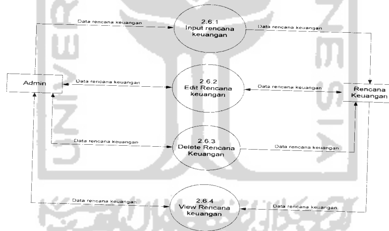
Gambar 3.11 DFD Level 3 proses manajemen data rencana keuangan
