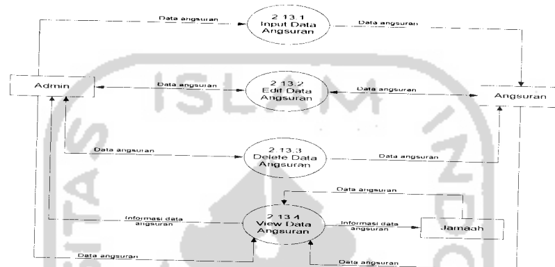
Gambar 3.17 DFD Level 3 proses manajemen data Angsuran
