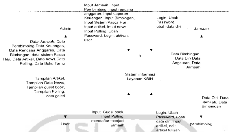
Gambar 3.1 Diagram Konteks (DFD Level 0)
