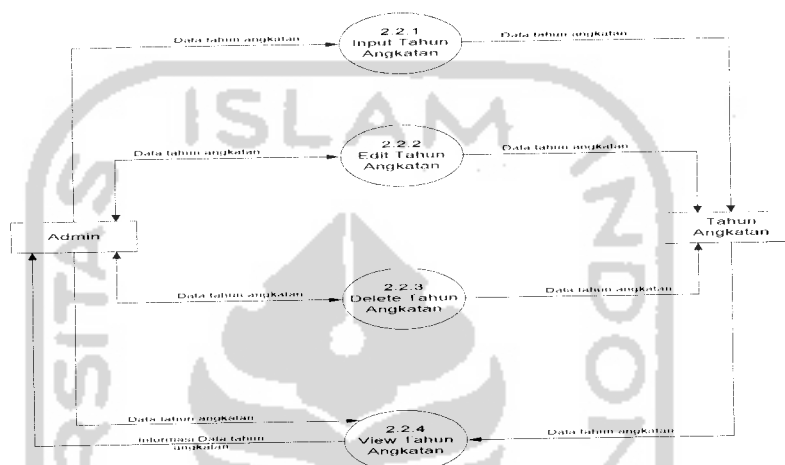
Gambar 3.7 DFD Level 3 proses manajemen data tahun angkatan
