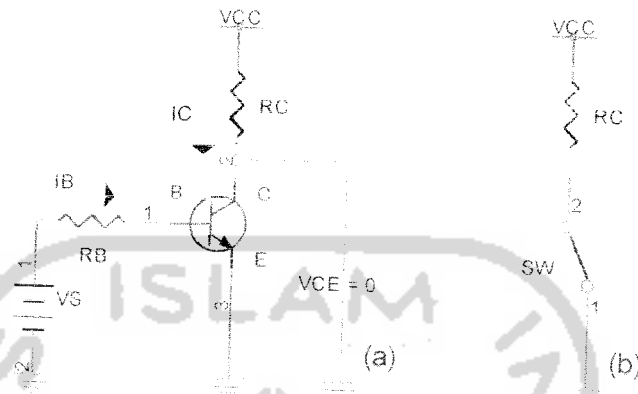
Gambar 2.8. (a) Transistor dalam keadaan konduktif. (b) Ekvivalen saklar tertutup
