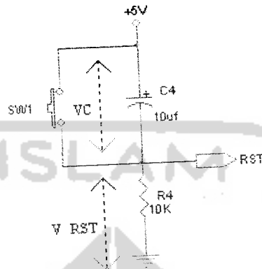
Gambar 4.3. Skema rangkaian reset
