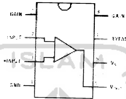
Gambar 2.4. IC LM 386
