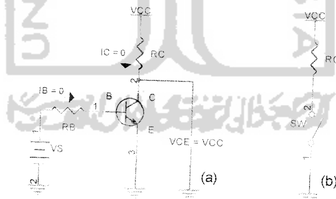
Gambar 2.9.(a) Transistor dalam keadaan non konduktif. (b) Ekvivalen saklar terbuka
