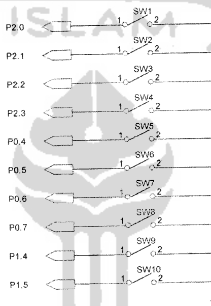
Gambar 3.5. Rangkaian micro switch
