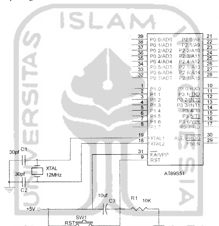
Gambar 3.4. Rangkaian sistem minimum mikrokontroller AT89S51
