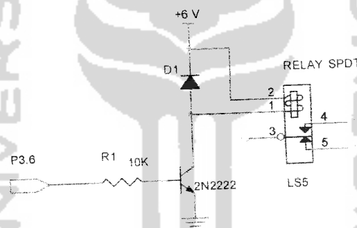
Gambar 4.4. Rangkaian pengujian penggerak relay
