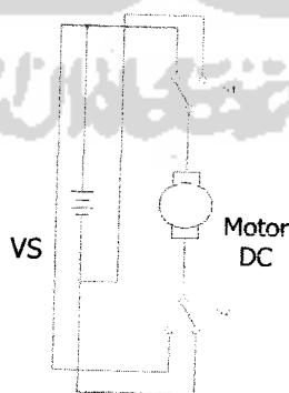
Gambar 2.12. Pengaturan arah motor dengan menggunakan saklar
