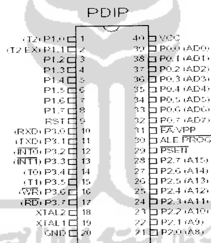
Gambar 2.1. Susunan kaki mikrokontroler AT89S51
