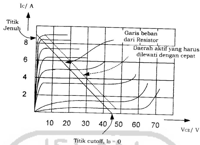
Gambar 2.7. Karakteristik beban DC Transistor (Sumber : Richard Blocher : 2003)
