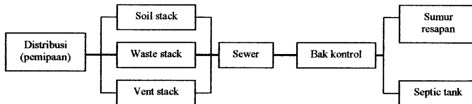
Gambar.IX.7.2 skema sistim sanitasi dan drainasi
