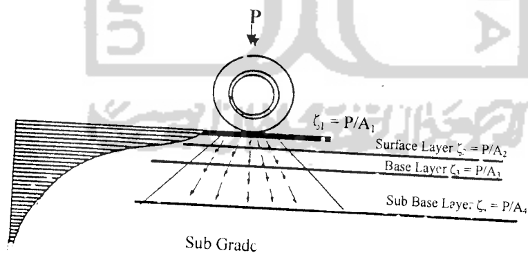
Gambar. 3.2 Penyebaran Beban Pada Masing-masing Lapis Perkerasan
