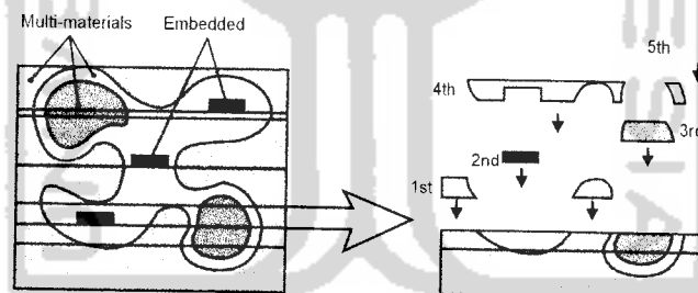
Gambar 2.8 (d) Struktur multi material dengan menyisipkan komponen [ http://www.cs.cmu.edu/~sdm/opener.htm ]
