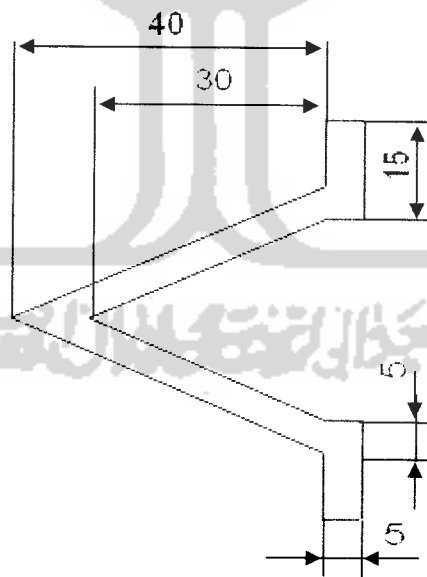
Gambar 4.28 Pola Lapisan ketiga dan kelima
