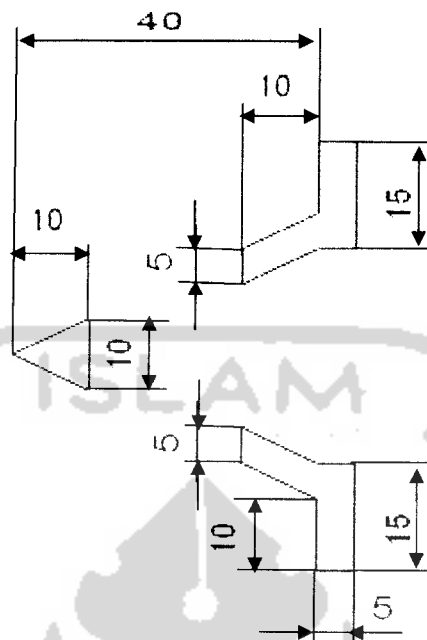
Gambar 4.28 Pola Lapisan ketiga dan kelima
