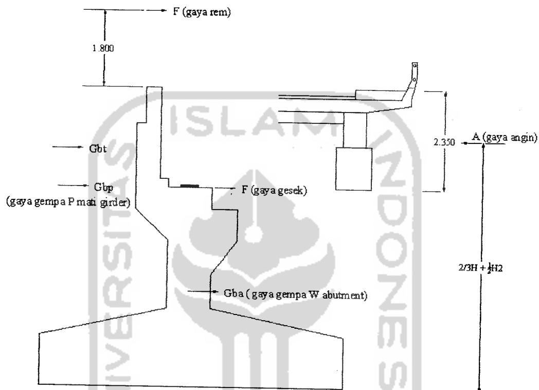
Gambar 3.18 Beban sekunder yang bekerja pada abutment
