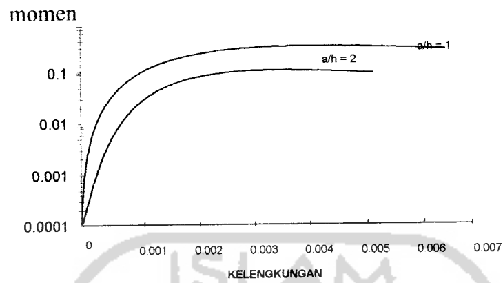
Gambar (3.21) Hubungan momen-kelengkungan
