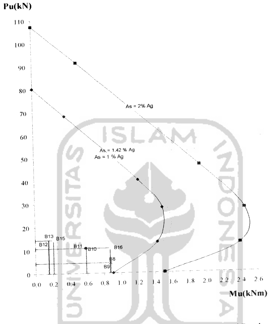
Gambar (5.13) Hubungan Mn-Pn Tinjauan Dimensi Batang Tepi Benda uji 2
