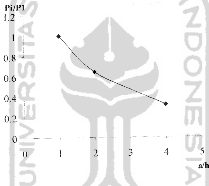
Gambar (5.9) Hubungan rasio a/h terhadap rasio pembebanan
