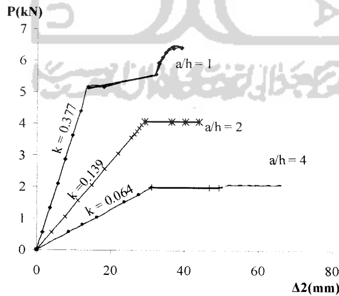
Gambar (5.4) Grafik regresi hubungan beban-deformasi pada \Delta 2
