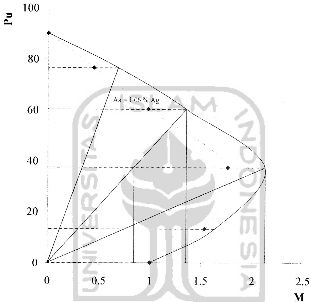
Gambar (5.15) Hubungan Mn-Pn Tinjauan Dimensi Batang Tepi Benda uji 3
