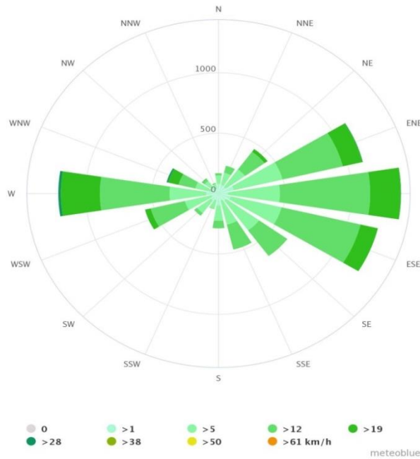
Data angin pada site
