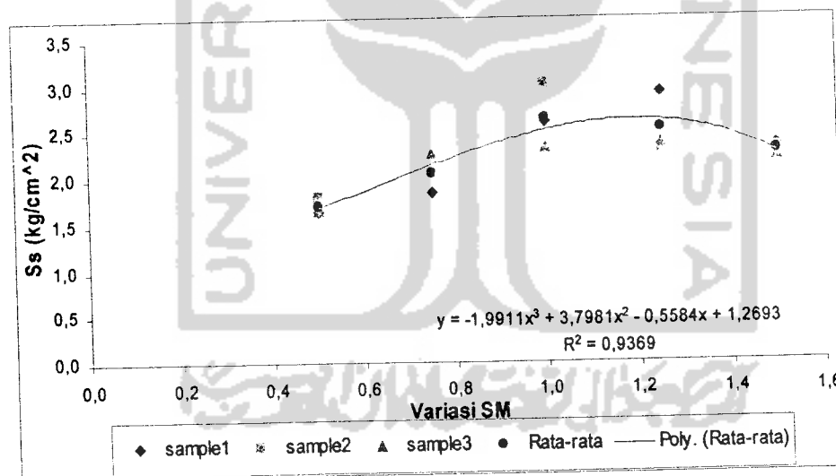
Gambar 5.6 Grafik Kuat Geser Pasangan Bata
