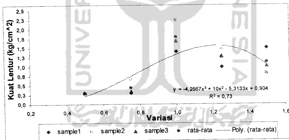
Gambar 5.4 Grafik Kuat Lentur Pasangan Bata
