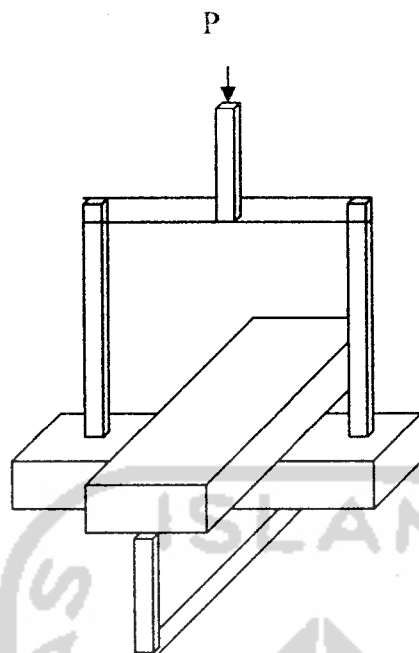
Gambar 4.3 Pengujian Lekatan Mortar
