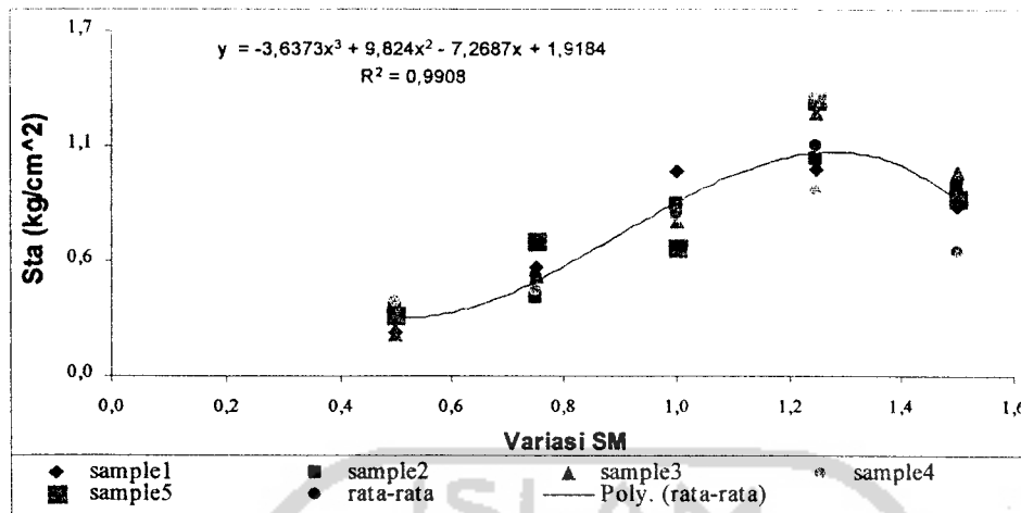
Gambar 5.2 Grafik Kuat Tarik Mortar
