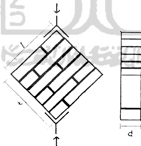
Gambar 4.8 Pengujian Kuat Geser Pasangan Bata Merah
