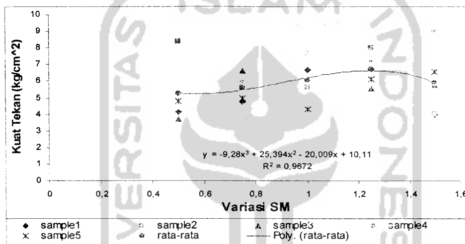
Gambar 5.1 Grafik Kuat Tekan Mortar
