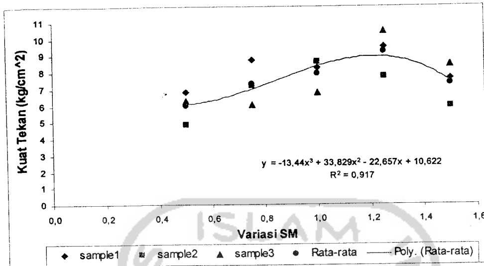
Gambar 5.5 Grafik Kuat Tekan Pasangan Bata
