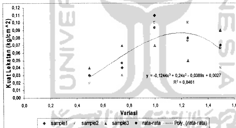
Gambar 5.3 Grafik Kuat Lekatan Mortar
