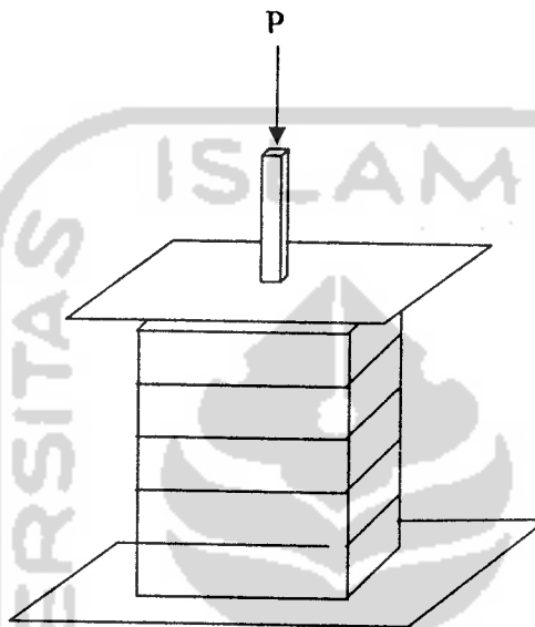
Gambar 4.7 Pengujian Kuat Tekan Pasangan Bata Merah
