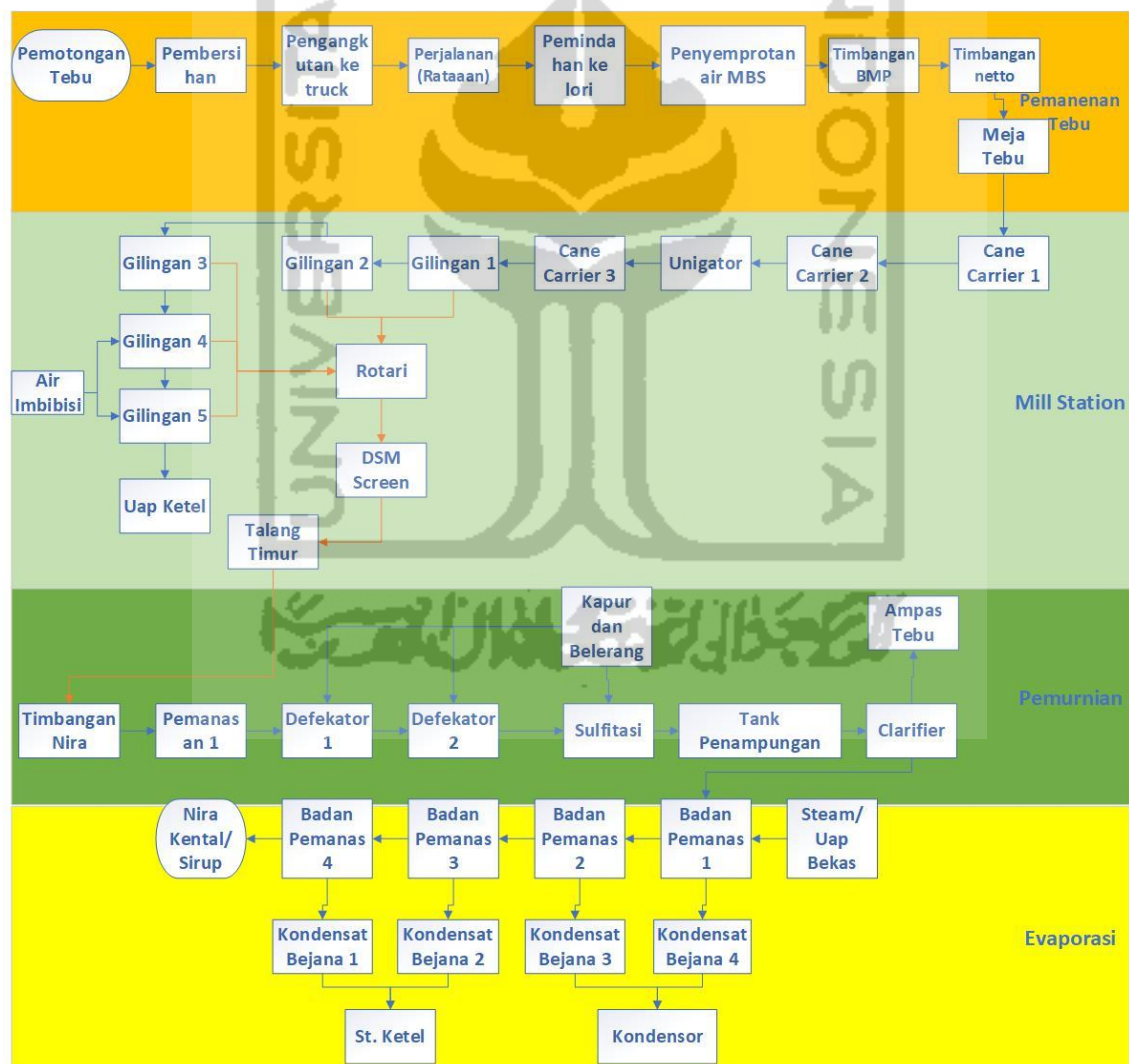
Gambar 4. 1 Flowchart pengolahan tebu sampai nira kental
