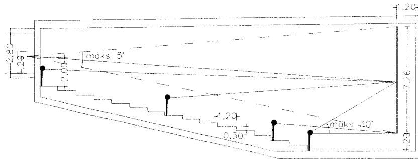
Jarak Pandang Penonton
