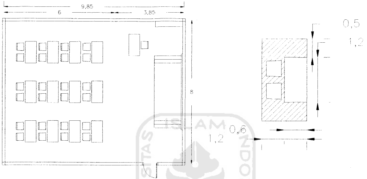
Layout R.Kelas
