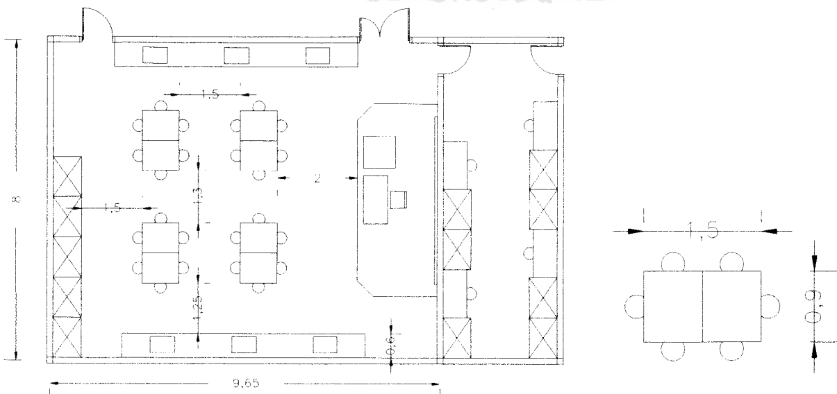
Layout R.Kelas
