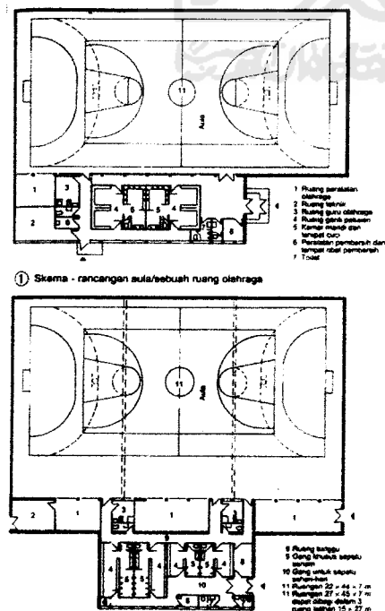
Lapangan Dengan Beberapa Fungsi
