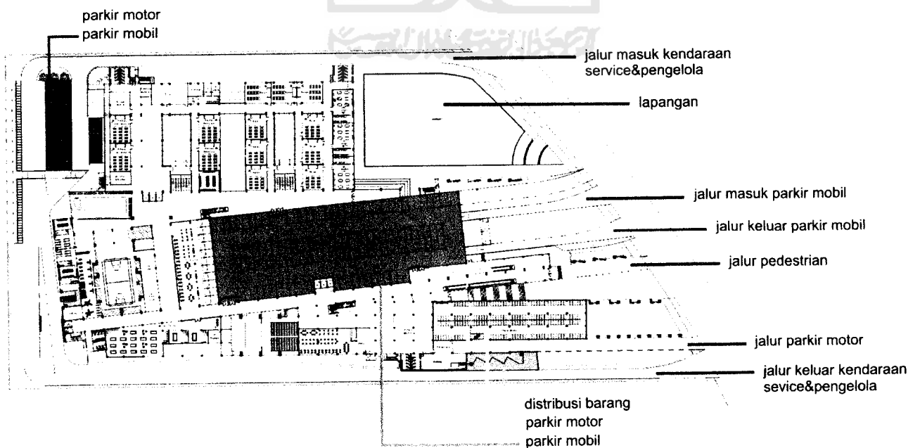
Tata Ruang Luar
