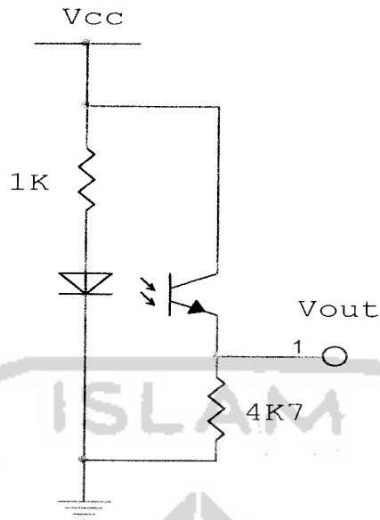
Gambar 2. 4 Rangkaian Optocoupler
