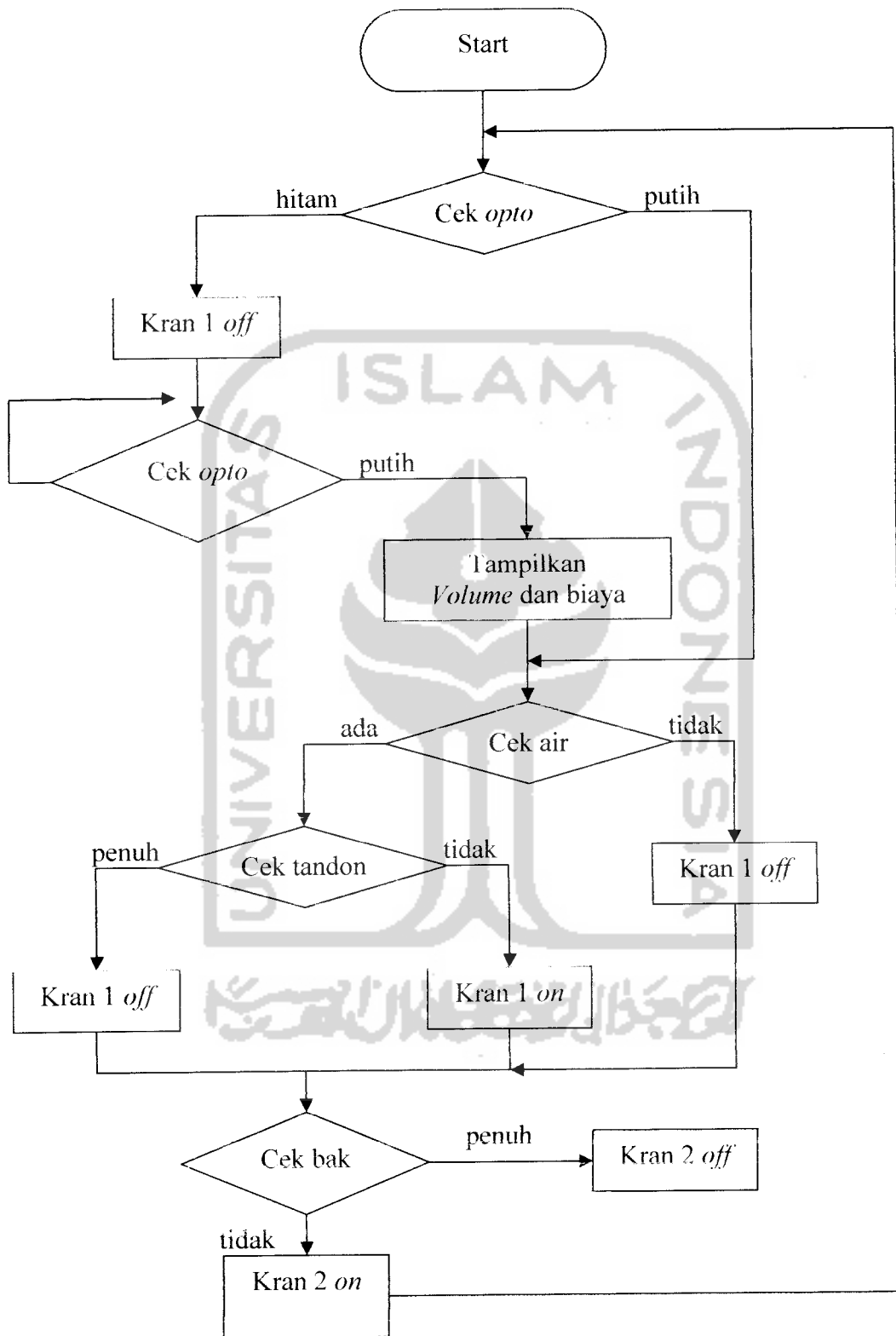
Gambar 3. 2 Diagram Alir Sistem
