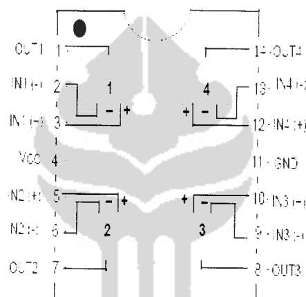
Gambar 2. 6 Konfigurasi Pin LM 324
