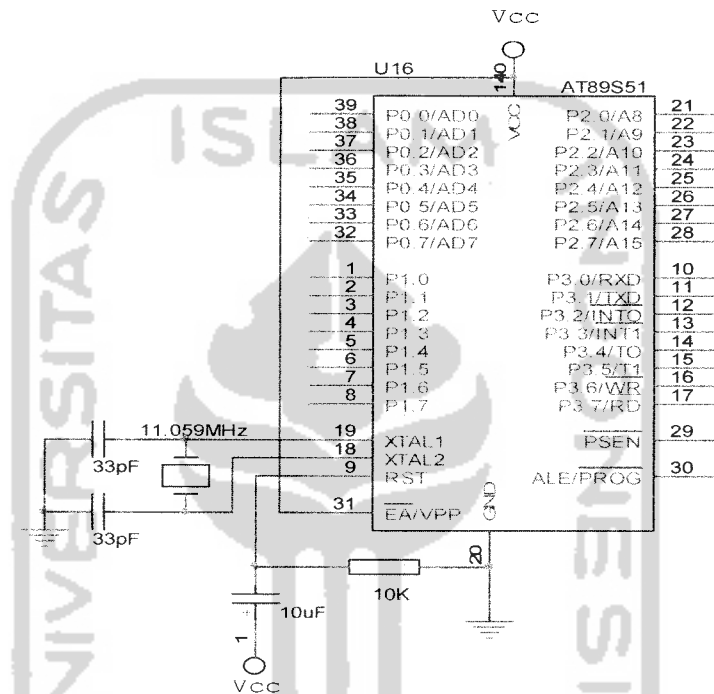
Gambar 3.9 Rangkaian Sistem Minimum AT89S51
