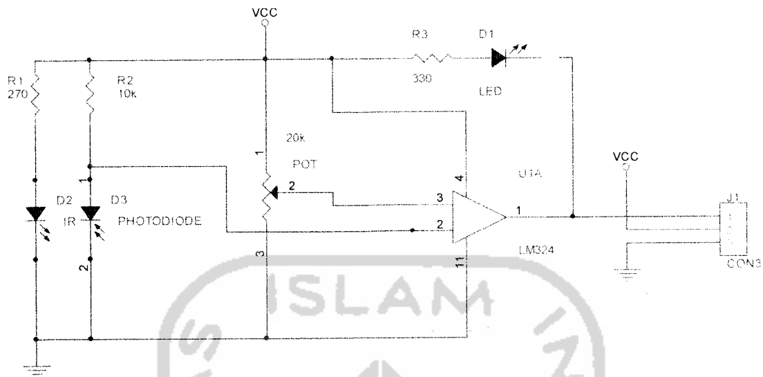
Gambar 3. 6 Rangkaian pembaca piringan kode
