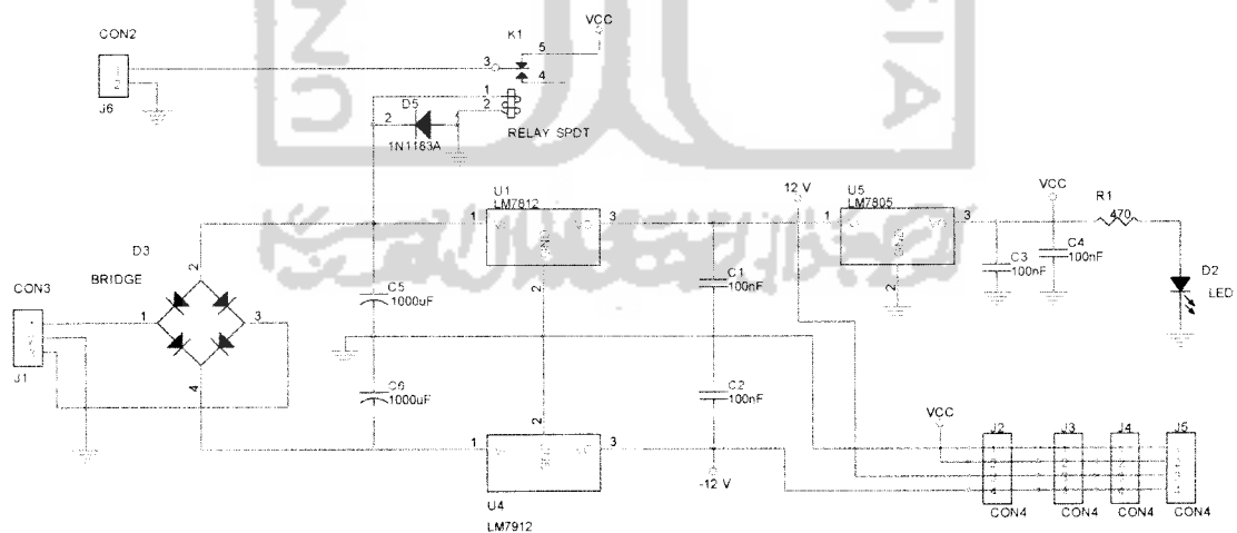
Gambar 3. 8 Rangkaian catu daya
