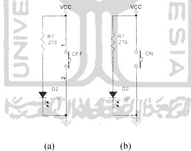
Gambar 3.5 Kondisi sensor optocoupler
