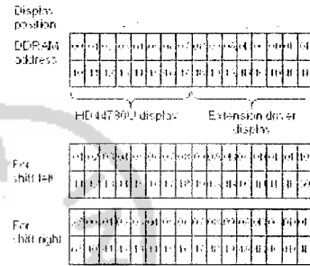
Gambar 1 DDRAM M1632 (diambil dari data sheet HD44780)
