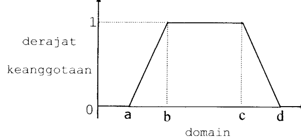
Gambar 2. 4 Kurva Trapesium
