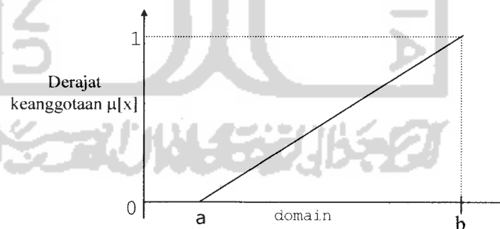
Gambar 2. 2 Representasi Linear Naik.
