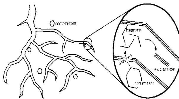
Gambar 2.4 Enzim yang memutus rantai karbon pada senyawa organik
