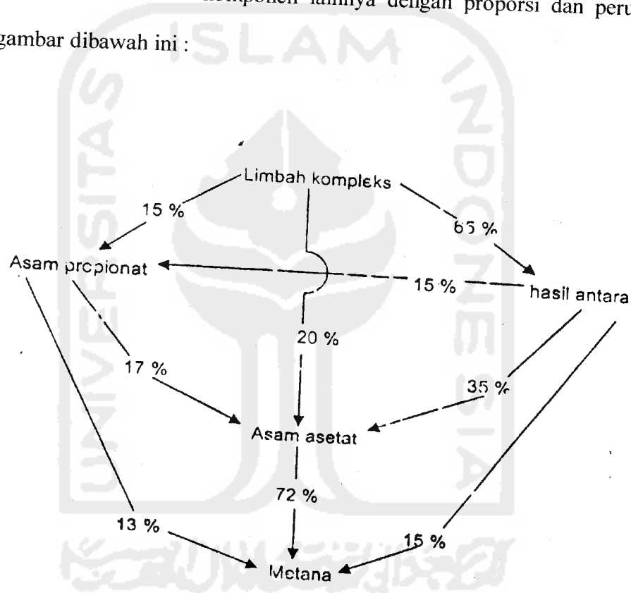
Gambar 3.1 Substrat dalam fermentasi anaerobik metana
