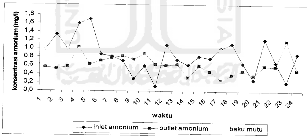
Gambar 5.20 Grafik perbandingan konsentrasi NH 3 (amoniak) dengan standar baku mutu
