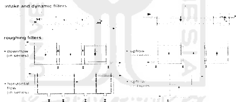
Gambar 2.4. Lay out umum dari Roughing Filter
