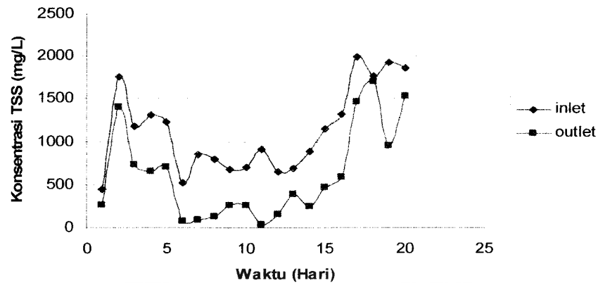
Gambar 4.3 Grafik Konsentrasi TSS pada Inlet dan Outlet
