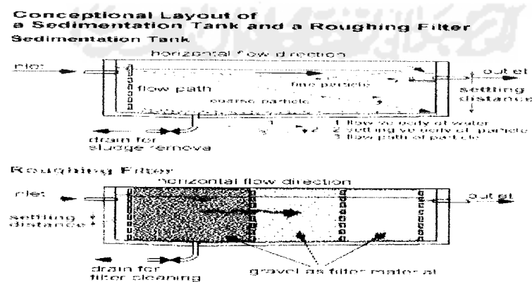
Gambar 2.3. Aplikasi dan konsep dari Roughing Filter
