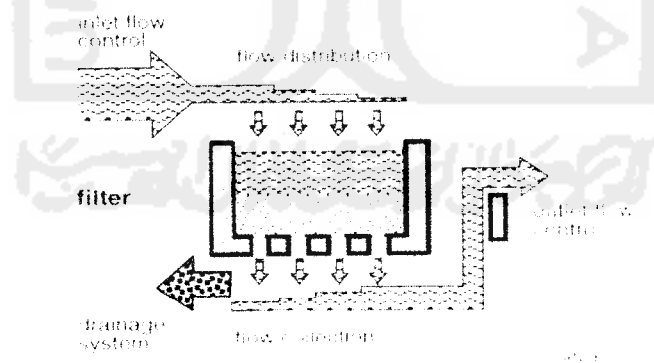
Gambar 2.5. Bagian Penting dari Roughing Filter
