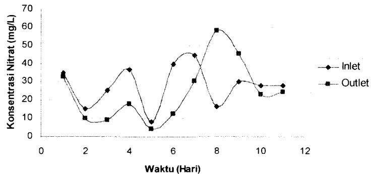
Gambar 4.1 Grafik Konsentrasi Nitrat pada Inlet dan Outlet
