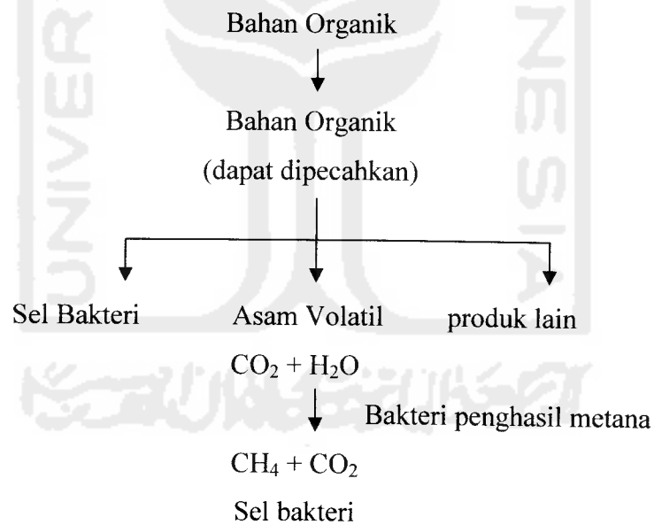
Gbr. 2.2. Mekanisme Pengolahan Anaerobik Air Limbah
