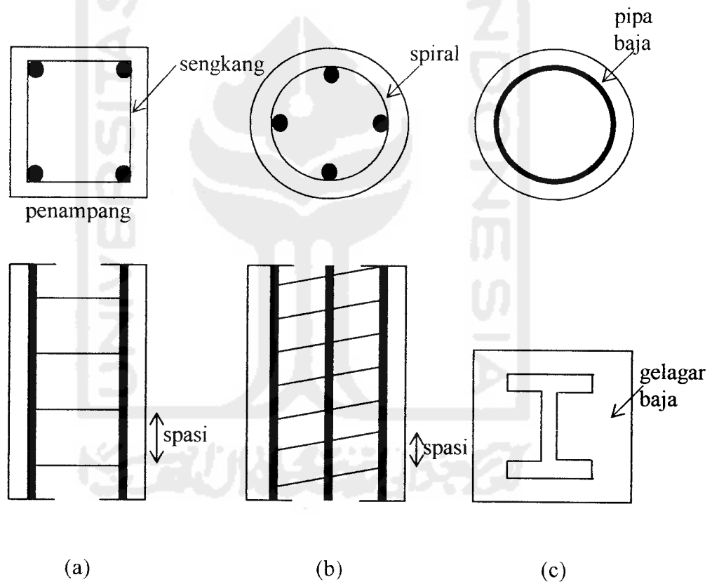
Gambar 2.1 Jenis-jenis kolom
