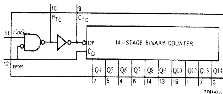
Gambar 2.8. Konfigurasi IC 4060
