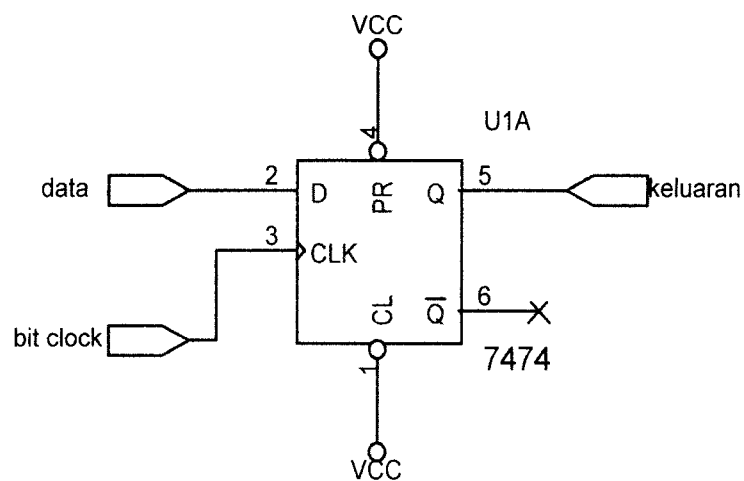
Gambar 3.4 Penyerempak data.
