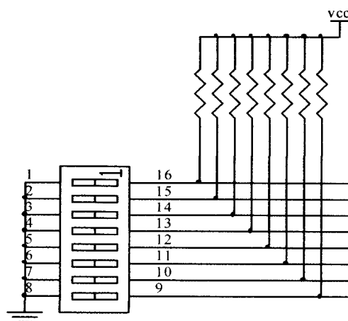
Gambar 3.2 Rangkaian DIP-Switch
