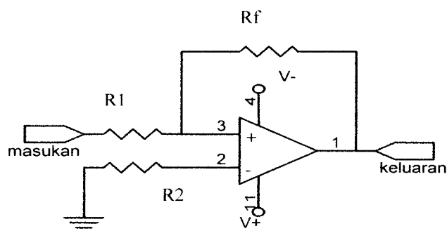
Gambar 3.10 Pembanding tegangan
