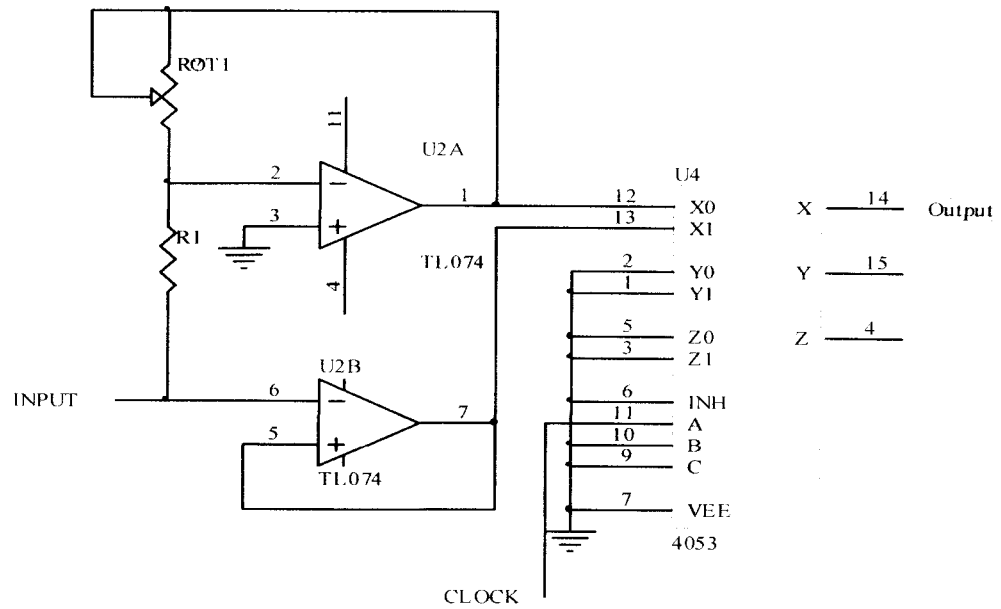
Gambar 3.7 Rangkaian demodulator
