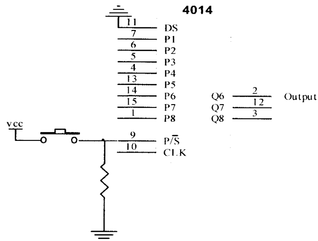
Gambar 3.3 Register geser paralel ke seri dengan masukan data 8-bit.
