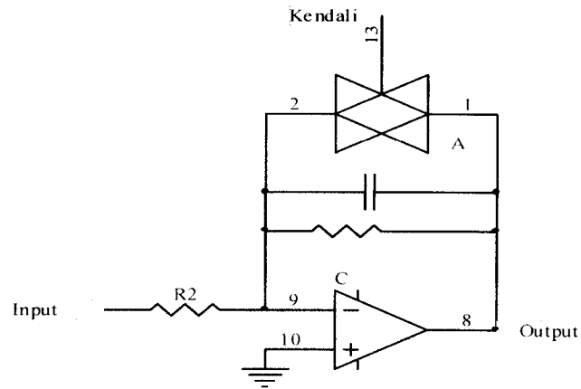
Gambar 3.9 Rangkaian pengintegral
