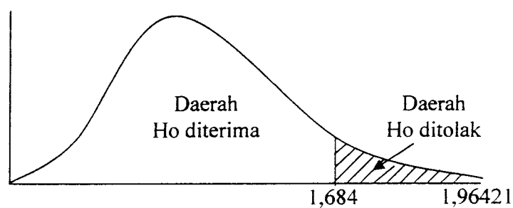
Kurva Uji t pendapatan konsumen
