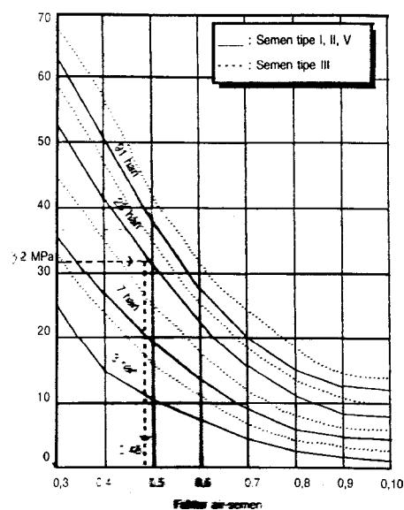
Gambar 3.1 Hubungan faktor air-semen dengan kuat tekan rata-rata
