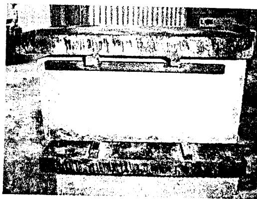
Gambar 21 Persiapan Pengujian Kuat Geser Beton
