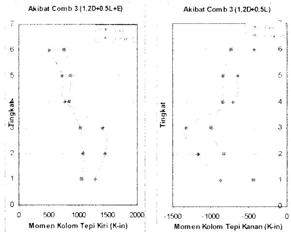
Grafik 6.31 Momen kolom Akibat Beban gravitasi+gempa Struktur 6 Lantai
