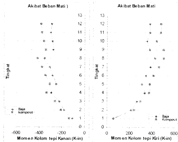
Grafik 6.20 Momen Kolom Akibat Beban Mati Struktur 12 Lantai
