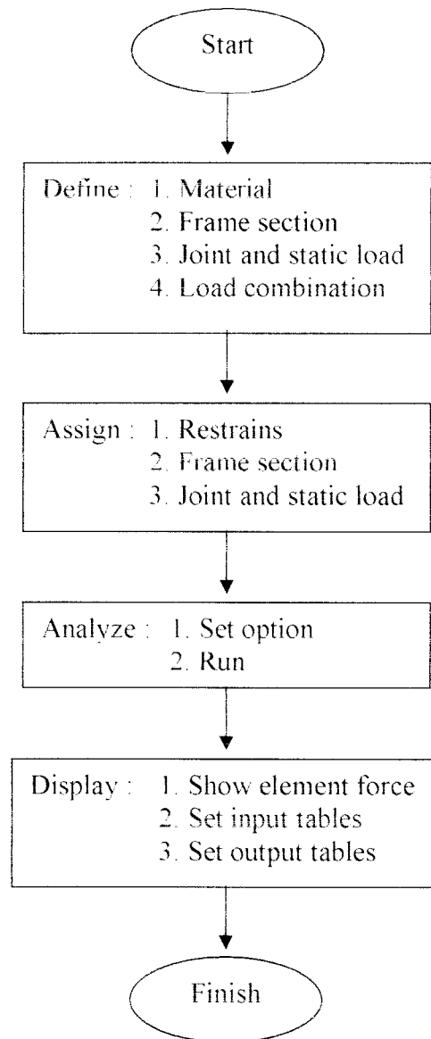
Gambar 4.7 Bagan alir analisis ETABS v.8.08.
