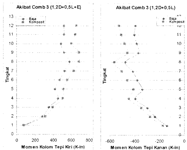
Grafik 6.32 Momen kolom Akibat Beban gravitasi+gempa Struktur 12 Lantai
