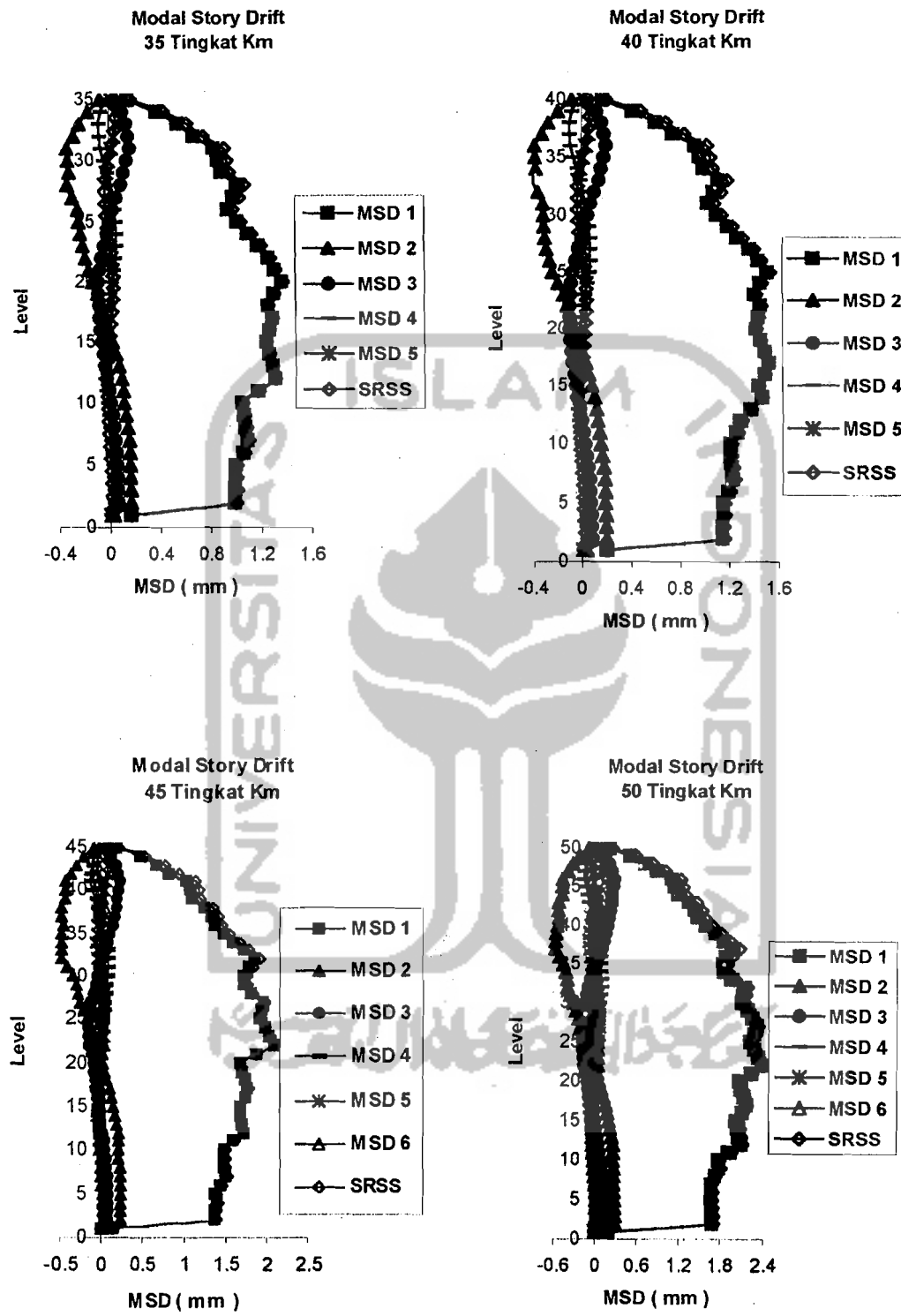
Gambar 5.11 Modal Story Drift untuk Muto
