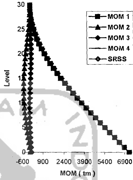
Modal Overtuning Moment 30 Tingkat Km
