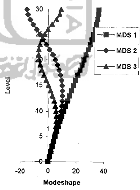
Modeshape 30 Tingkat Kf
