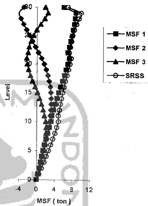
Modal Seismic Force 30 Tingkat Kf
