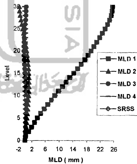
Modal Lateral Displacement 30 Tingkat Km
