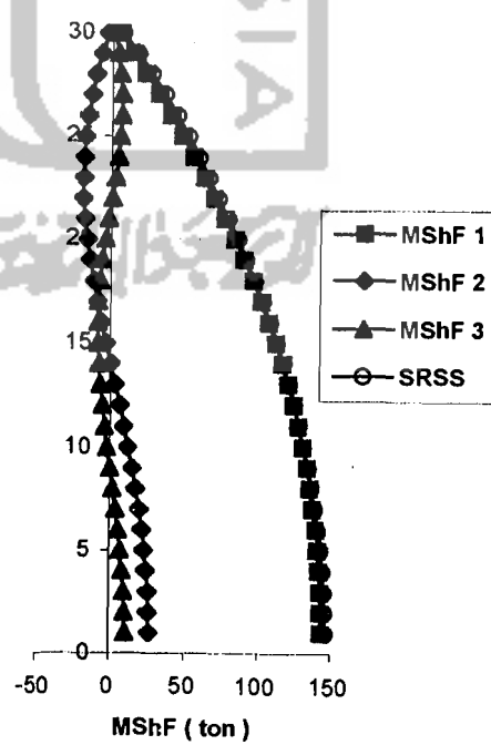
Modal Shear Force 30 Tingkat Kf
