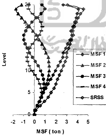
Modal Seismic Force 25 Tingkat Km
