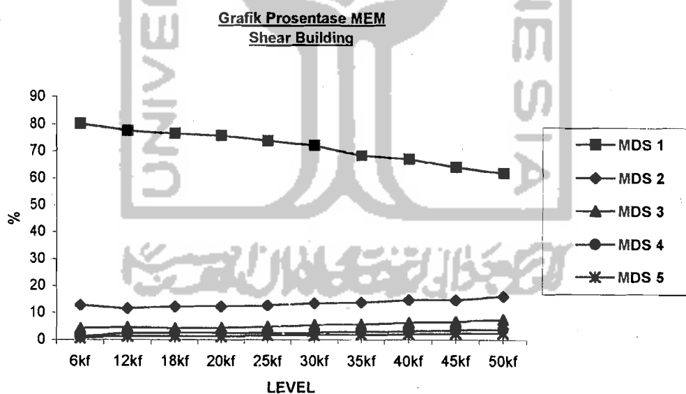
Gambar 5.24 Grafik % Modal Effective Mass untuk Shear Building
