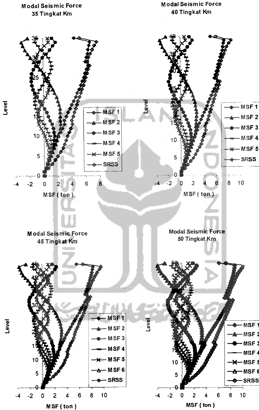
Gambar 5.5 Modal Seismic Force untuk Muto
