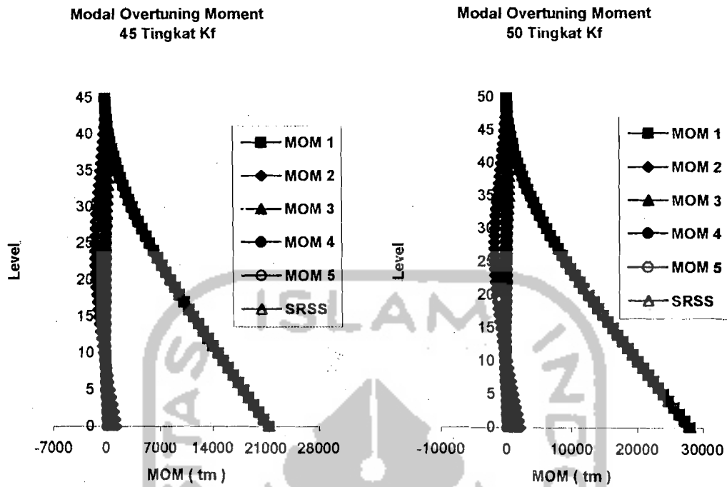
Gambar 5.8 Modal Overtuning Moment untuk Shear Building
