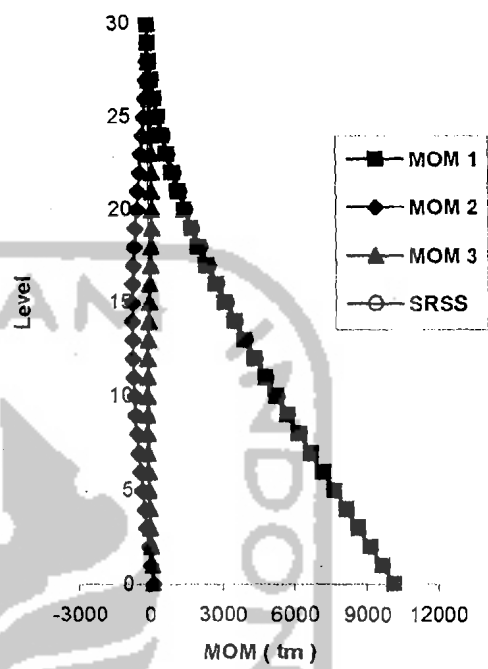
Modal Overtuning Moment 30 Tingkat Kf
