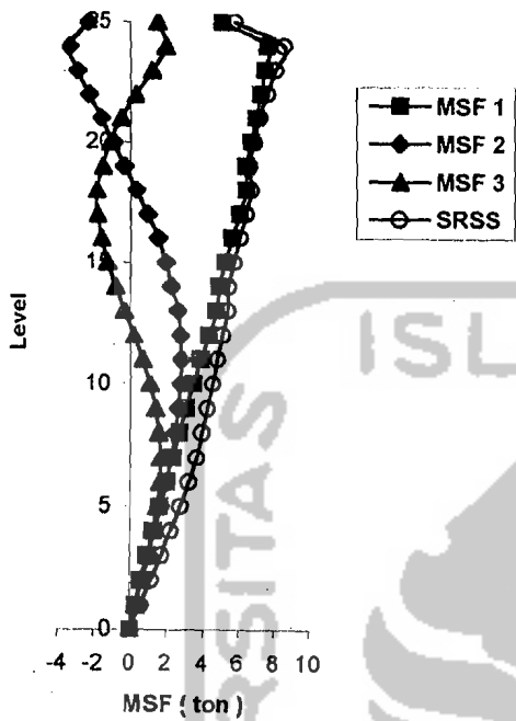
Modal Seismic Force 25 Tingkat Kf
