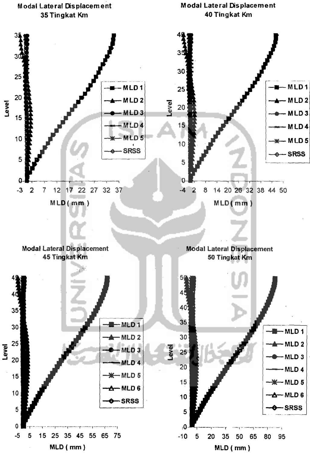
Gambar 5.13 Modal Lateral Displacement untuk Muto
