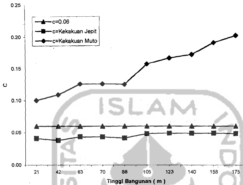
Gambar 5.21 Grafik Perbandingan Koefisien C
