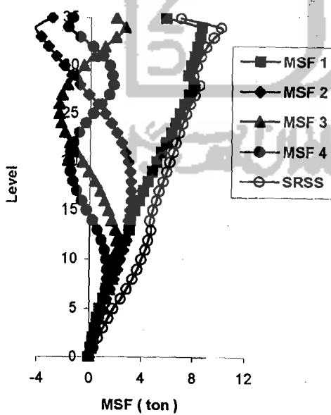
Modal Seismic Force 35 Tingkat Kf
