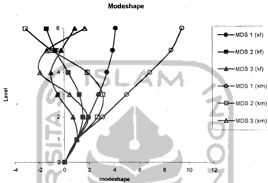
Gambar 5.30 Perbandingan Modeshape struktur 6 Tingkat
