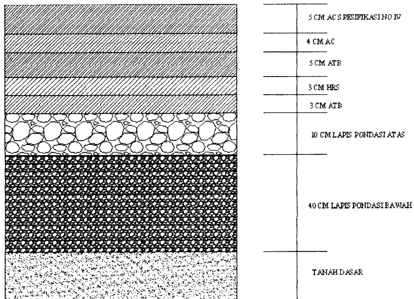
Gambar 5.10 Perancangan Tebal Lapis Tambahan ( Overlay )
