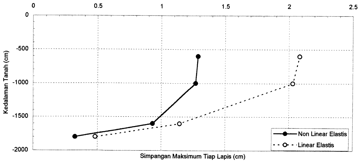
Grafik 6.15. Perbandingan Simpangan Tanah Non Linier Elastis dan Linier Elastis Dengan Massa Bangunan 40000 ton Pada Lapis Teratas Untuk Data Tanah Tawang Sari I Sukoharjo Akibat Gempa El Centro
