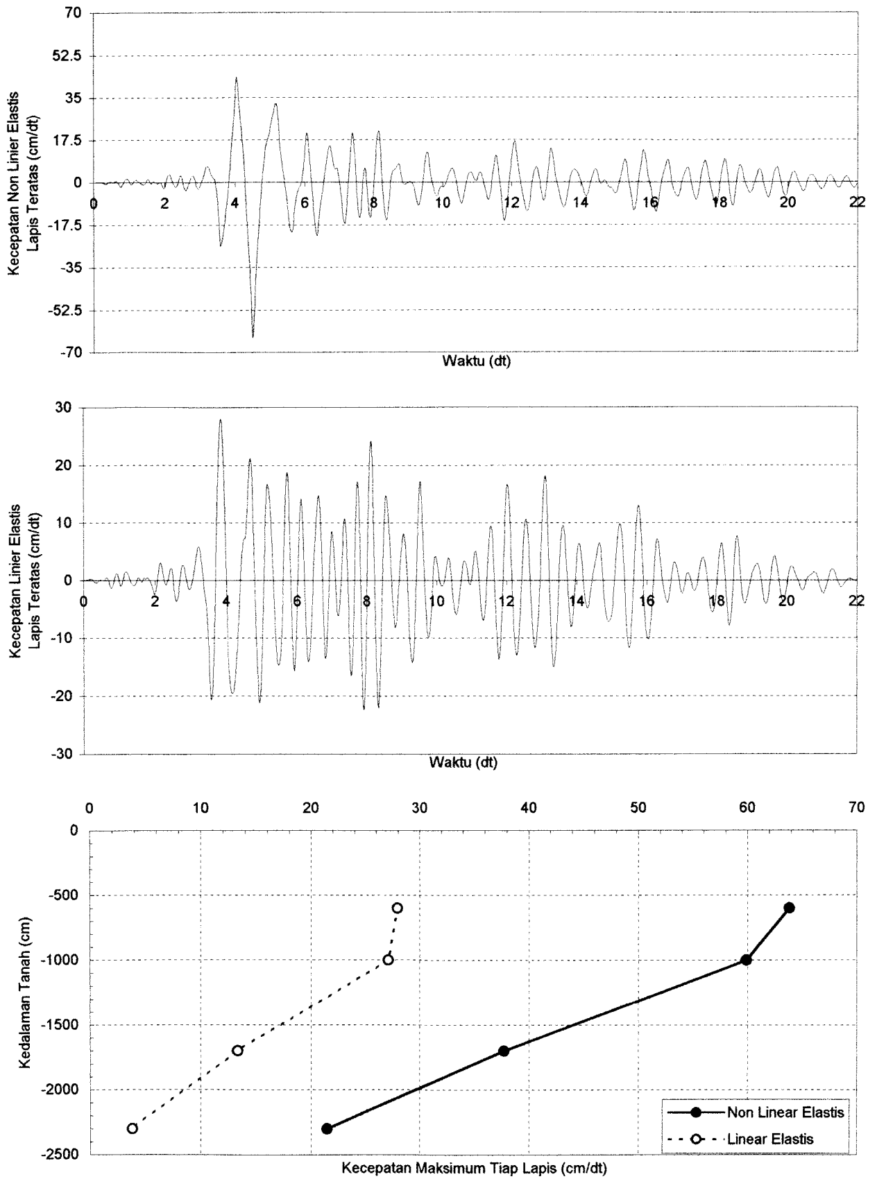
Grafik 6.120. Perbandingan Kecepatan Tanah Non Linier Elastis dan Linier Elastis Dengan Massa Bangunan 20000 ton Pada Lapis Teratas Untuk Data Tanah Tawangarsi II Sukoharjo Akibat Gempa Kobe
