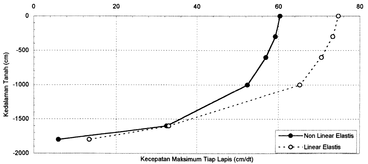
Grafik 6.42. Perbandingan Kecepatan Tanah Non Linier Elastis dan Linier Elastis Tanpa Massa Bangunan Pada Lapis Teratas Untuk Data Tanah Tawang Sari I Sukoharjo Akibat Gempa Kobe
