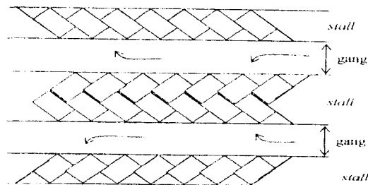
Gambar 3.10 Pola Parkir Tulang Ikan Tipe A
