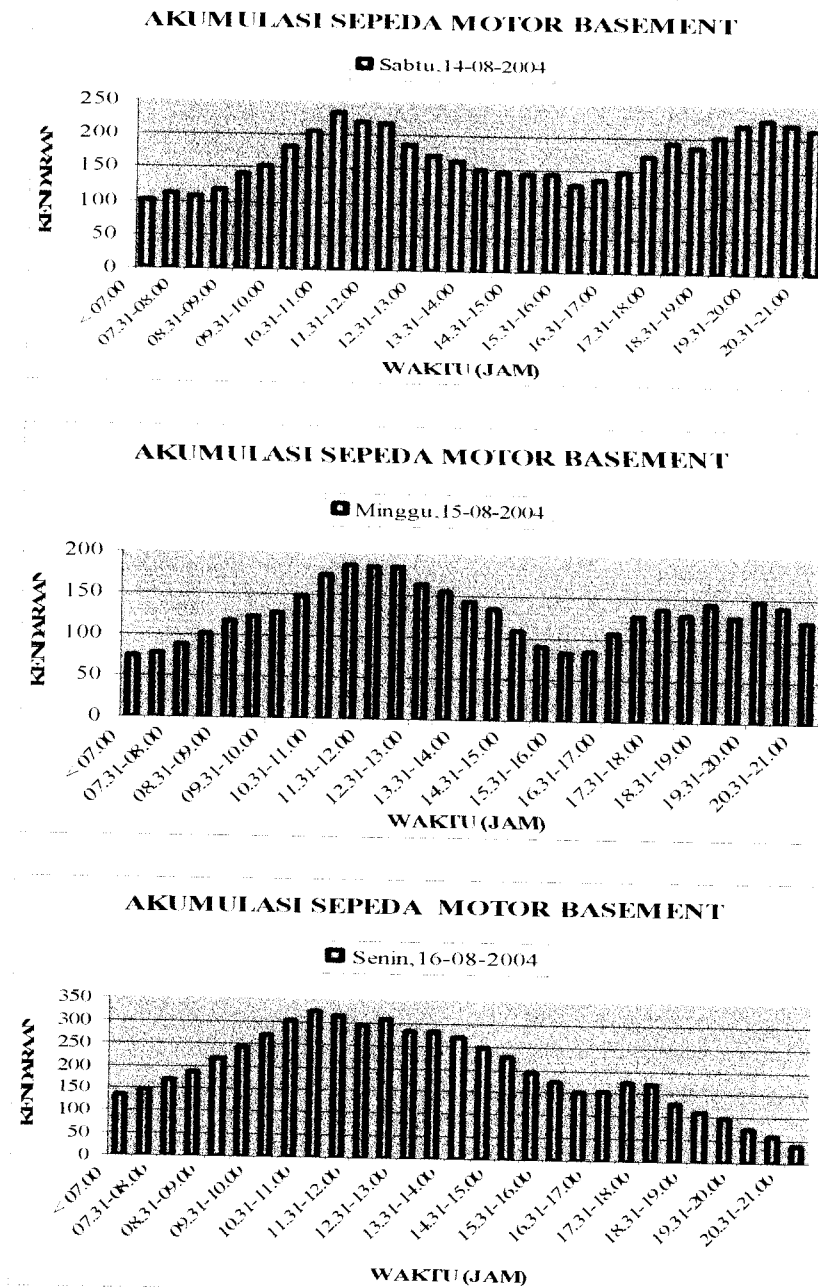
Gambar 5.9 Grafik Akumulasi Parkir Sepeda Motor Basement Selama Tiga Hari Sumber: Pengolahan Data, 2004
