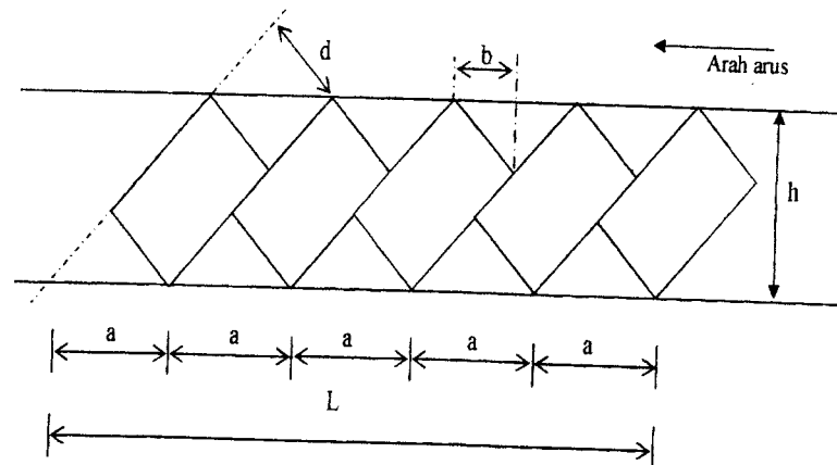
Gambar 5.11 Sketsa Ruang Parkir
