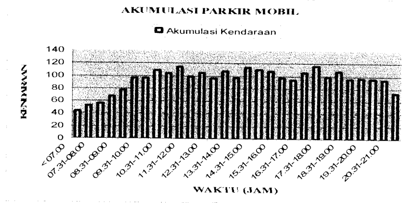
Gambar 5.7 Grafik Akumulasi Parkir Mobil Tanggal 16 Agustus 2004 Sumber: Pengolahan Data, 2004
