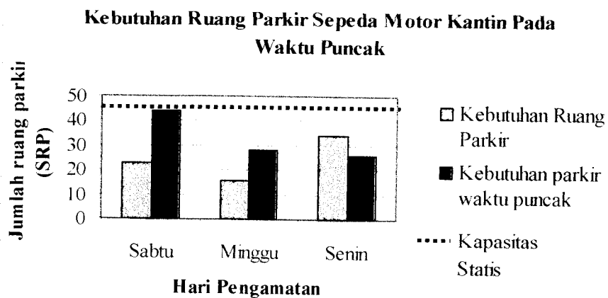
Gambar 5.14 Kebutuhan Ruang Parkir Sepeda Motor Kantin Pada Waktu Puncak Sumber : Pengolahan Data, 2004
