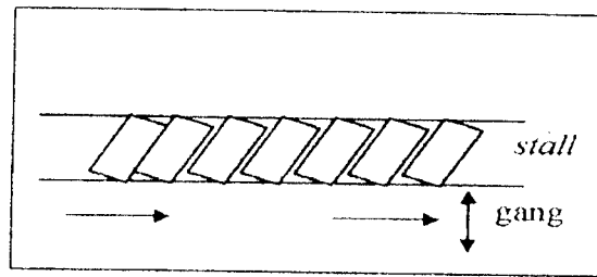
Gambar 3.6 Pola Parkir Satu Sisi Sudut 30^\circ , 45^\circ , 60^\circ
