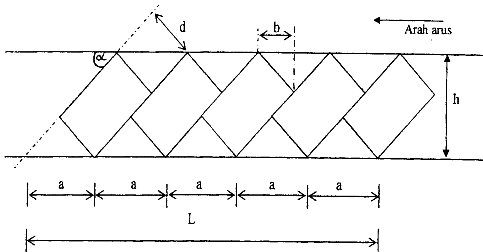
Gambar 3.13 Sketsa Ruang Parkir
