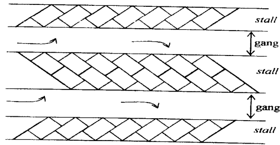
Gambar 3.12 Pola Parkir Tulang Ikan Tipe C
