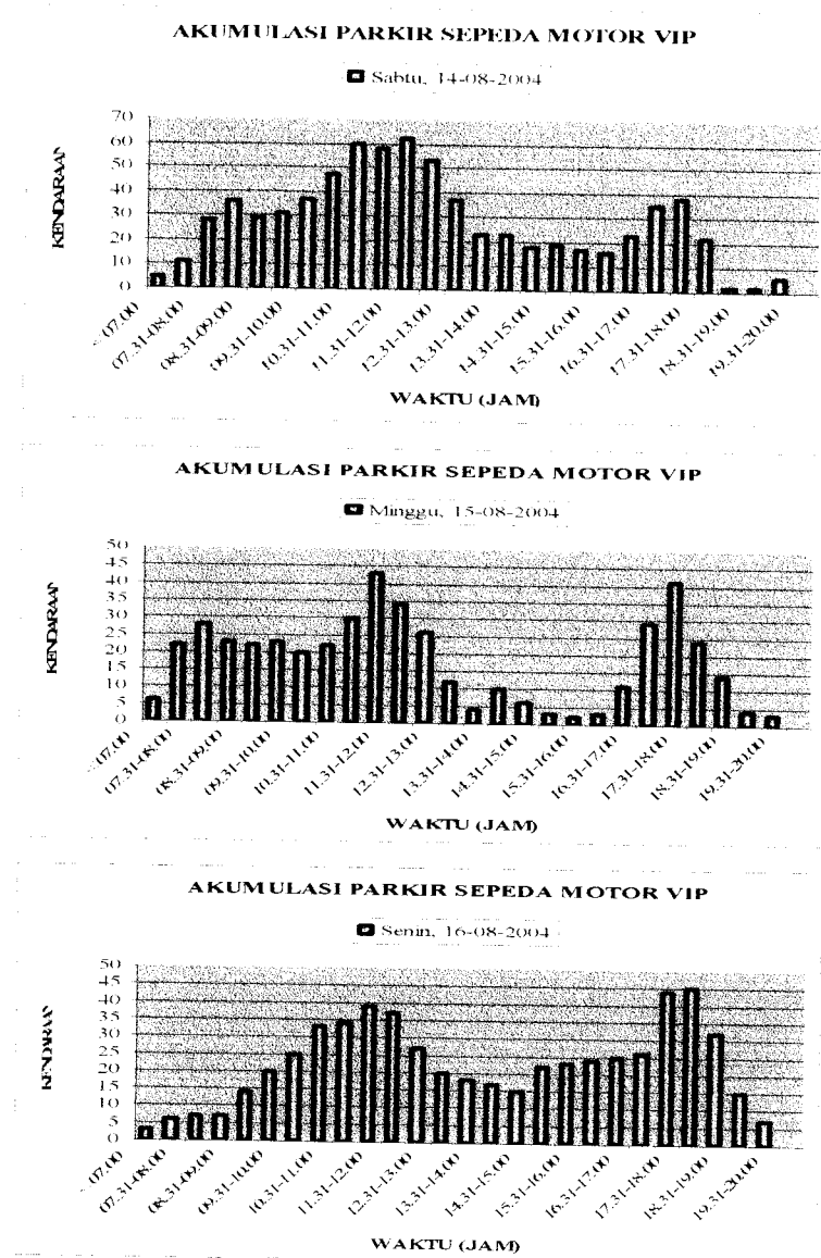
Gambar 5.8 Grafik Akumulasi Parkir Sepeda Motor VIP Selama Tiga Hari Sumber: Pengolahan Data, 2004
