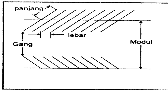
Gambar 3.18 Ukuran Pelataran Parkir Sudut
