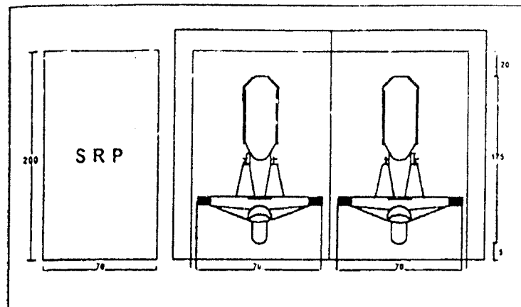
Gambar 3.3 Satuan Ruang Parkir Untuk Sepeda Motor (dalam cm) Sumber: Departemen Perhubungan 1996
