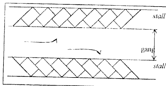
Gambar 3.8 Pola Parkir Dua Sisi Sudut 30^\circ , 45^\circ , dan 60^\circ
