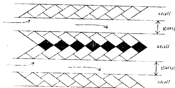
Gambar 3.11 Pola Parkir Tulang Ikan Tipe B
