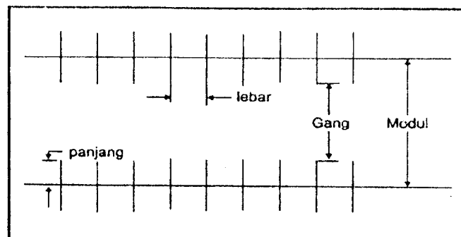
Gambar 3.17 Ukuran Pelataran Parkir Tegak Lurus
