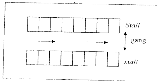
Gambar 3.7 Pola Parkir Dua Sisi Sudut 90^\circ
