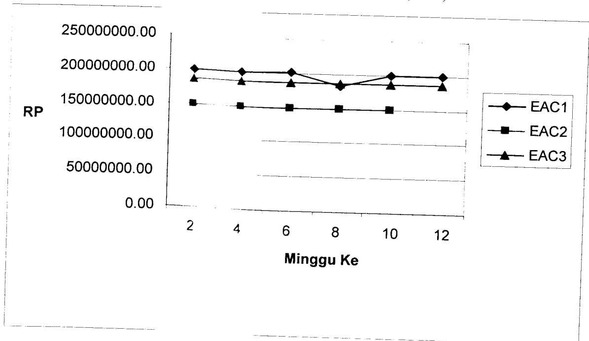
Gambar 6.5. Grafik Nilai Perkiraan Biaya Total (EAC)
