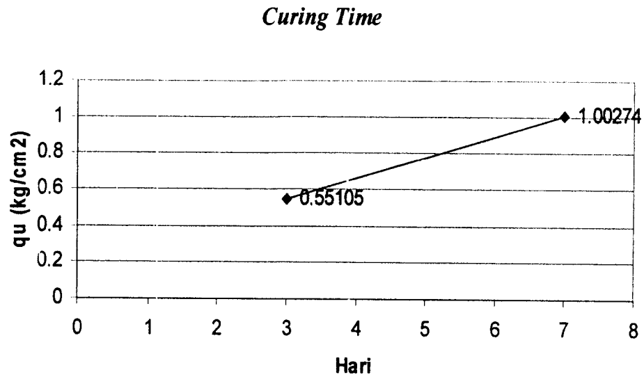
Gambar 6.3 Grafik Nilai qu pada uji tekan bebas dengan Curing Time pada kadar campuran kapur tumbuk 10 %
