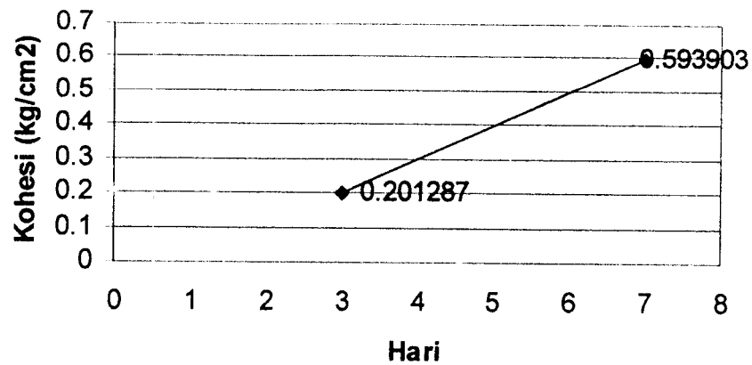
Gambar 6.7 Grafik Nilai Kohesi dengan Curing Time Uji Triaksial UU pada Kadar Campuran Kapur Tumbuk 10%
