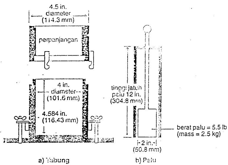
Gambar 3.9 Alat uji Proctor Standar : (a) cetakan, (b) penumbuk
