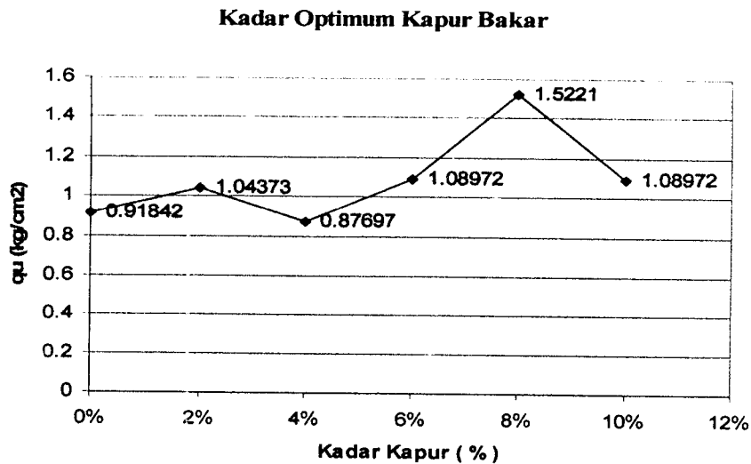
Gambar 6.2 Grafik hasil Uji Gambut + Kapur Bakar pada Uji Tekan Bebas
