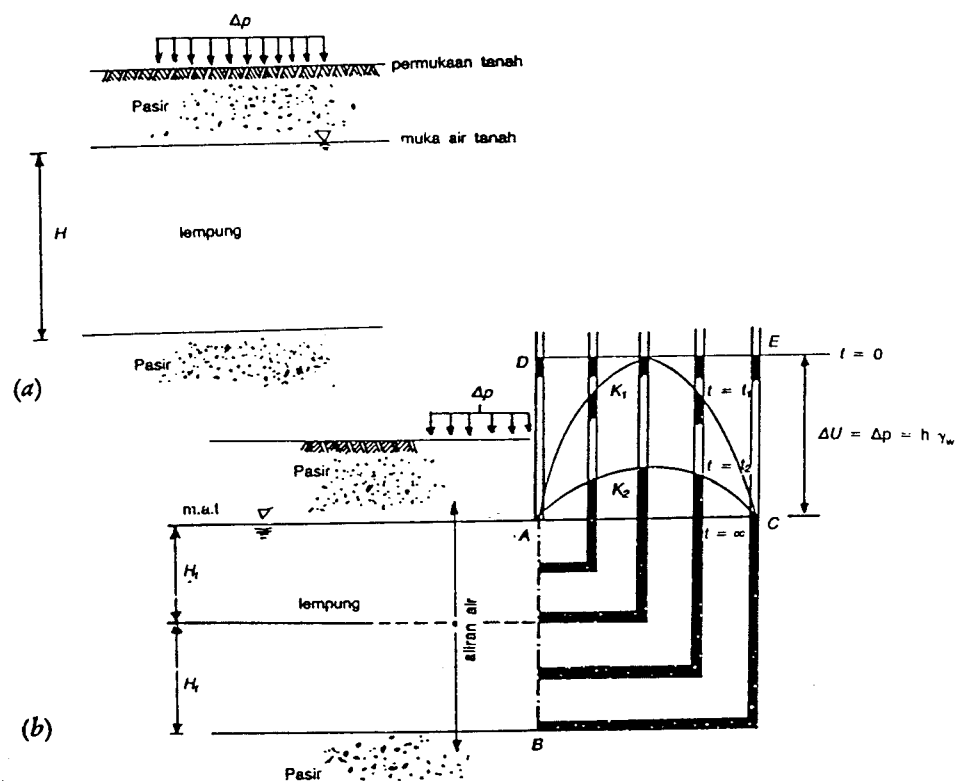
Gambar 3.19 Reaksi tekanan air pori terhadap beban pondasi
