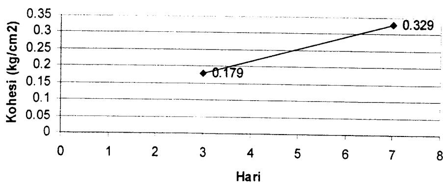
Gambar 6.5 Grafik Nilai Kohesi pada Uji Tekan Bebas dengan Curing Time pada kadar campuran kapur tumbuk 10%
