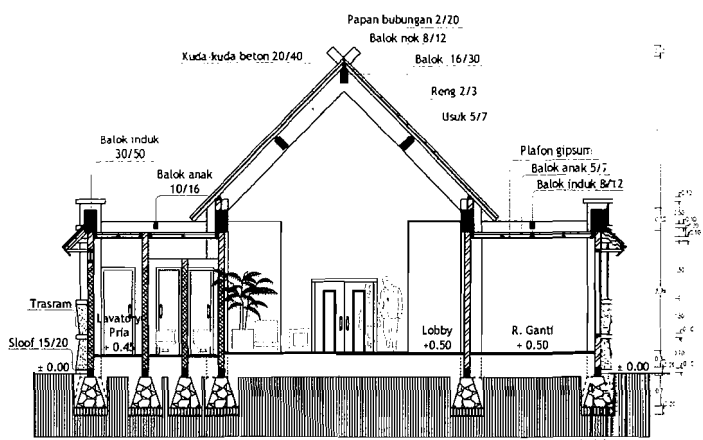
Potongan A-A Zone 3
