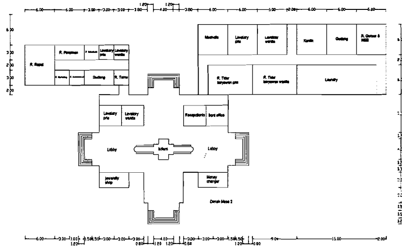
Denah Masa Lobby Zone 2 & Pengelola
