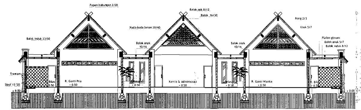
Potongan A-A Zone 3 Fasilitas Olahraga
