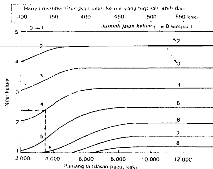
Gambar 3.1 'Nilai Keluar' Untuk Jalan Keluar Yang Tegak Lurus
