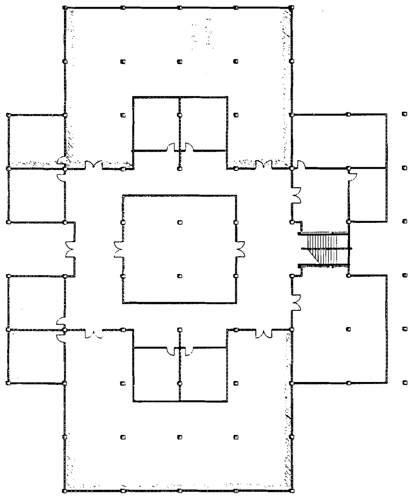
LANTAI SATU
