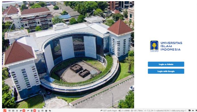
Gambar 4. 1 Halaman Login
