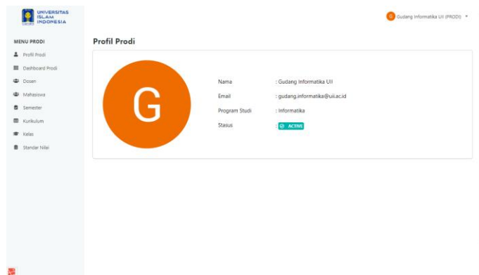
Gambar 4. 6 Halaman Profil
