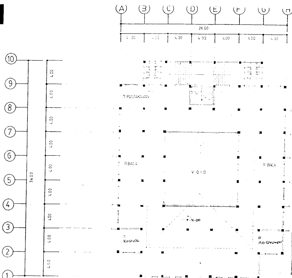
DENAH PERPUSTAKAAN LT.02
