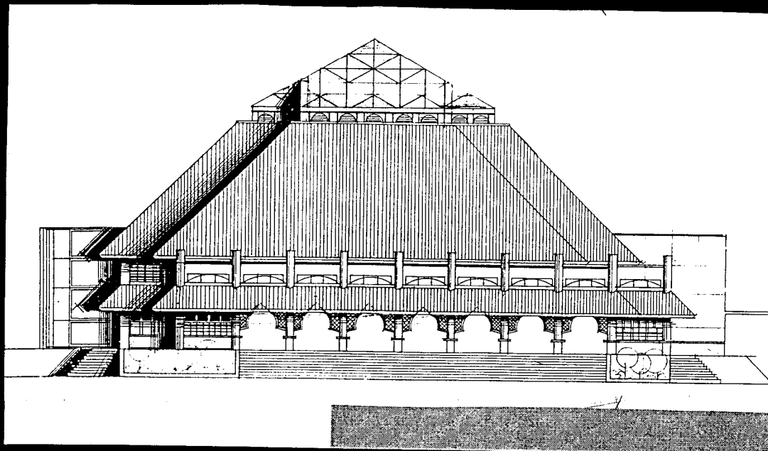
TAMPAK SELATAN
