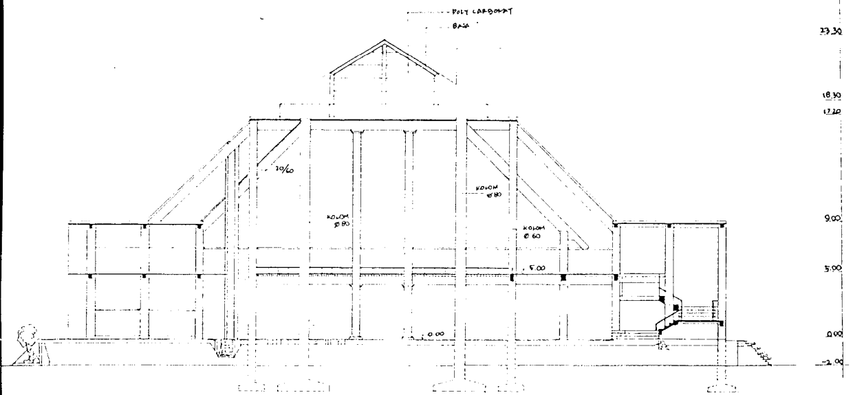
POTONGAN MASJID
