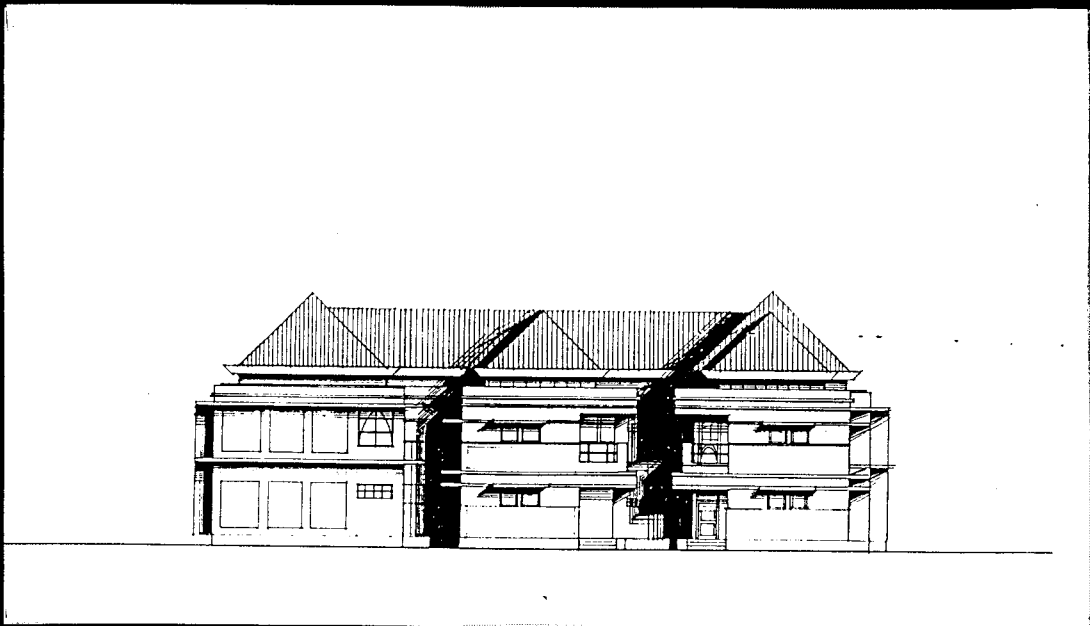
TAMPAK TIMUR
