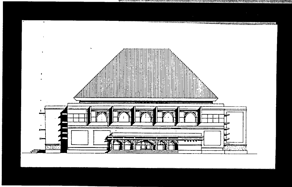
TAMPAK SELATAN
