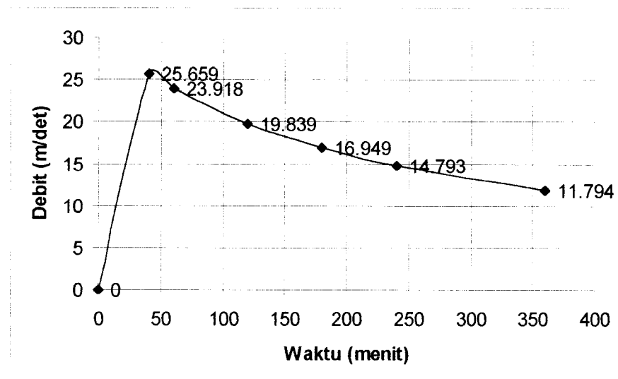
Grafik 5.10 Hidrograf Aliran Limpasan Permukaan Periode Ulang 10 Tahunan
