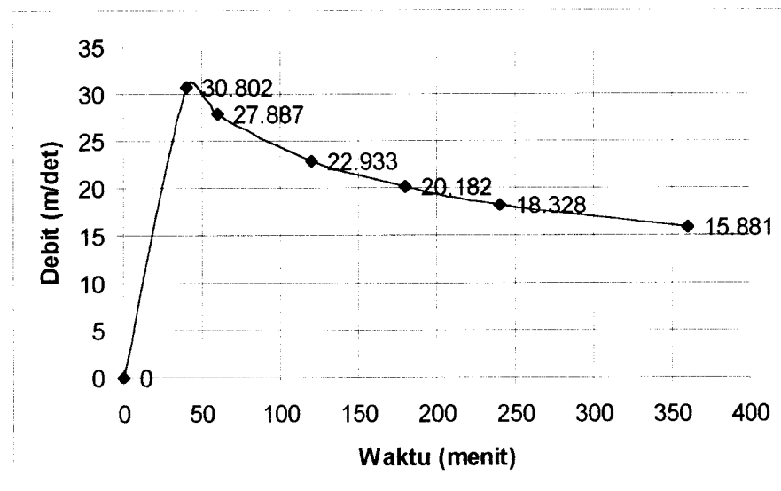
Grafik 5.11 Hidrograf Aliran Limpasan Permukaan Periode Ulang 20 Tahunan
