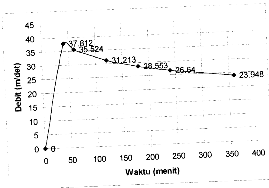
Grafik 5.13 Hidrograf Aliran Limpasan Permukaan Periode Ulang 100 Tahunan
