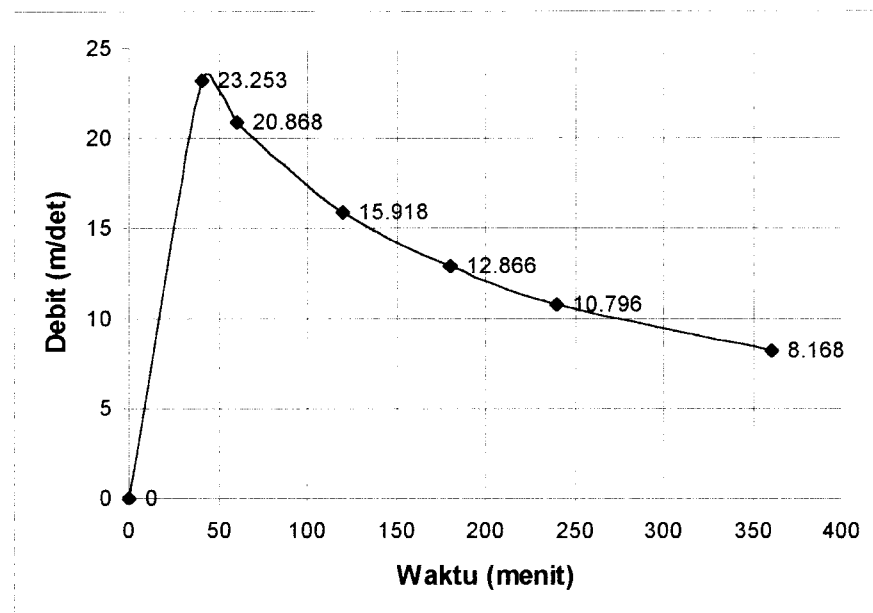
Grafik 5.9 Hidrograf Aliran Limpasan Permukaan Periode Ulang 5 Tahunan
