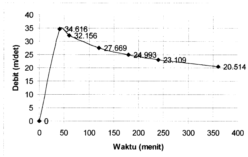
Grafik 5.12 Hidrograf Aliran Limpasan Permukaan Periode Ulang 50 Tahunan
