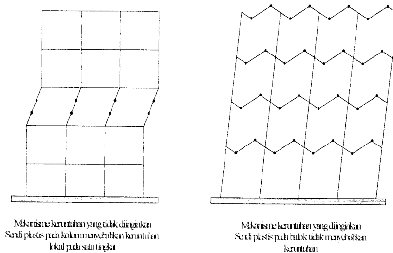
Gambar 3.1. Mekanisme khas yang dapat terjadi pada portal rangka terbuka
