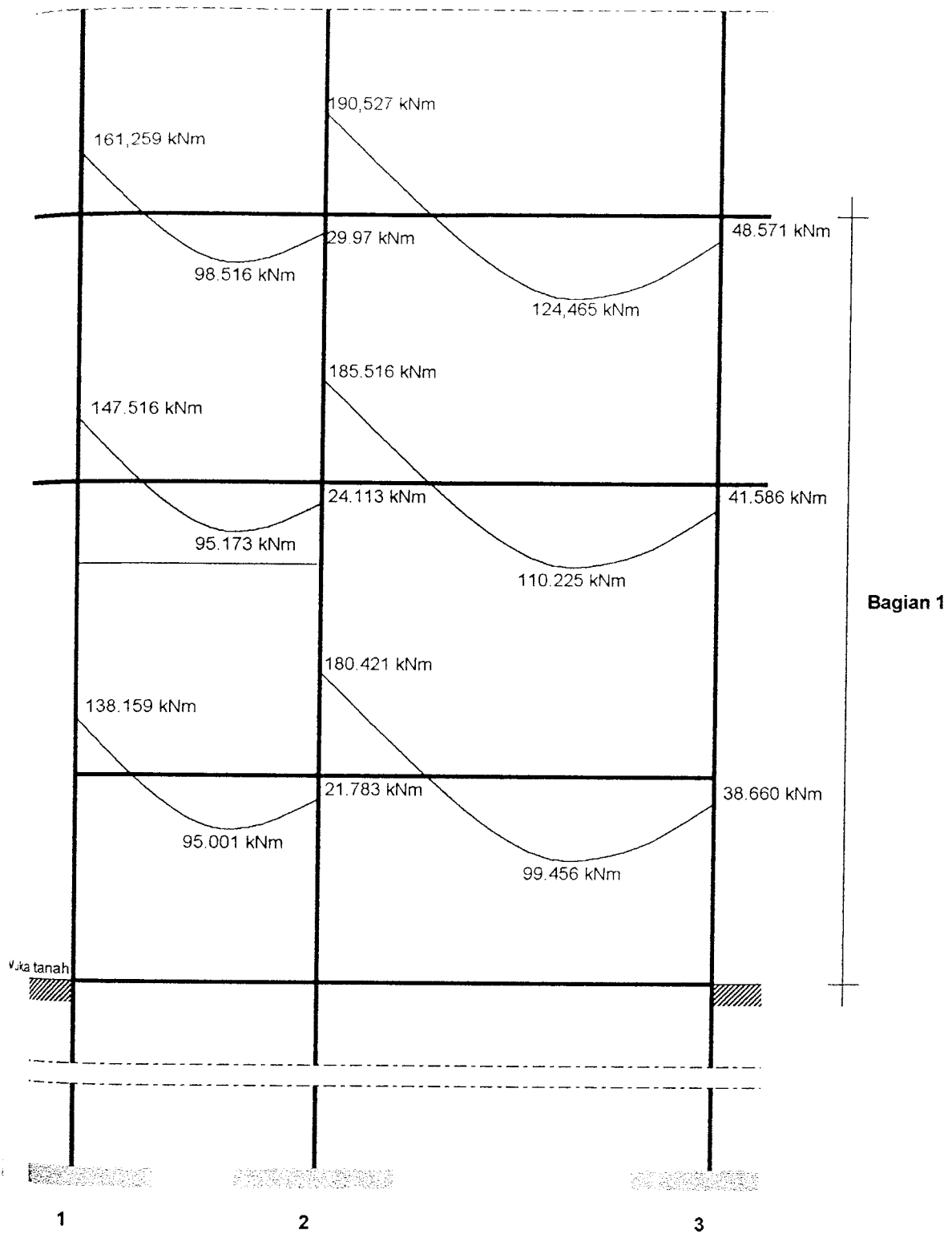
Gambar diagram momen akibat kombinasi beban 0,9 M_D \pm M_{E,K}
