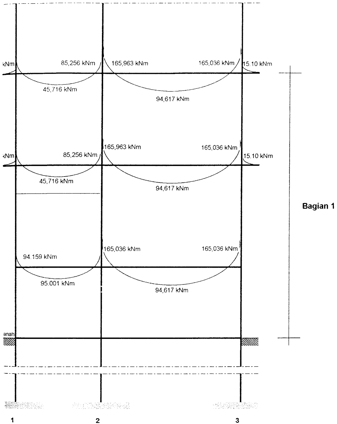
Gambar diagram momen akibat kombinasi beban 1,2 MD + 1,6 ML
