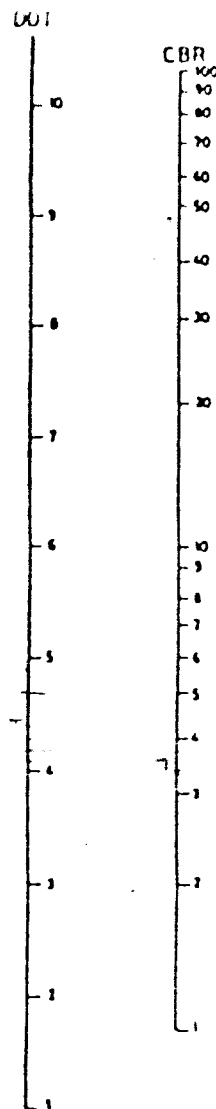
Gambar 1 KORELASI DDT DAN CBR
