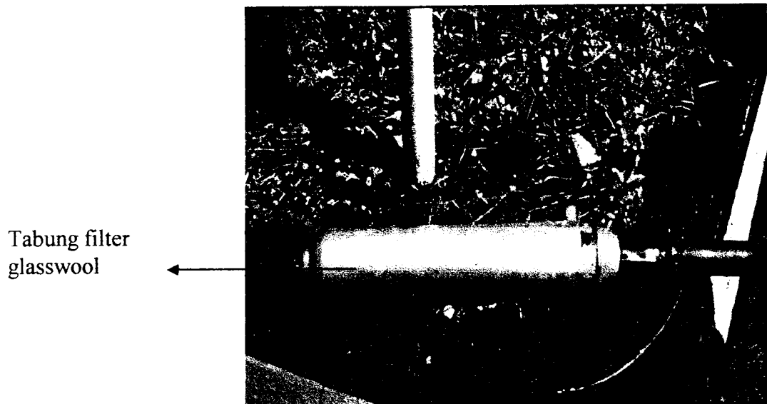
Gambar 3.6 Pemasangan adaptor dengan tabung filter glasswool
