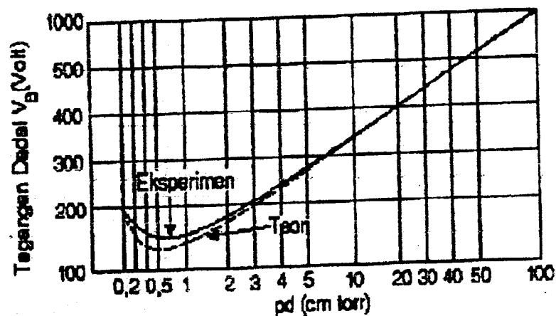
Gambar 2.2 Kurva Paschen
