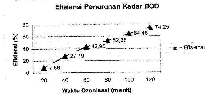
Grafik Efisiensi Penurunan Kadar BOD
