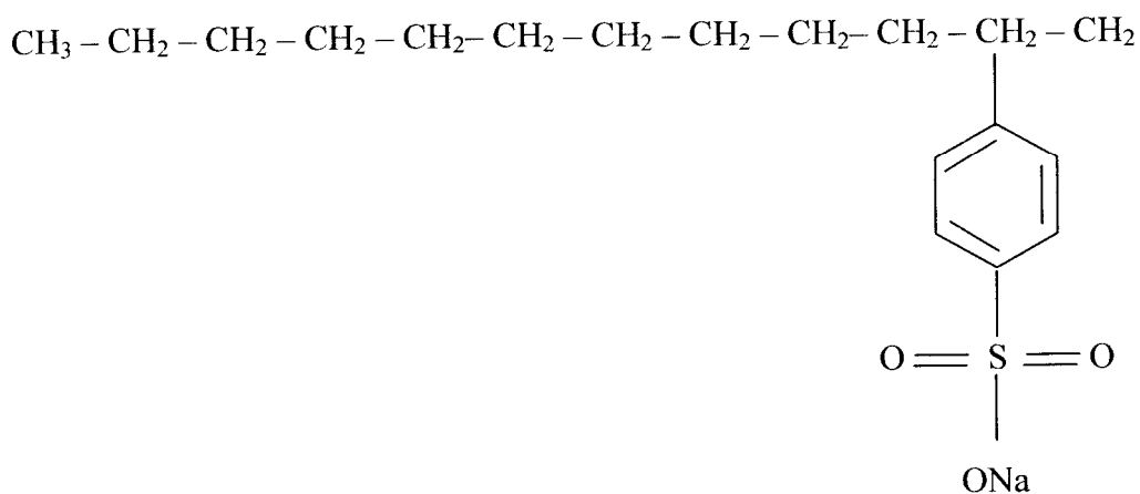
Gambar 4.11 Rumus Struktur Diterjen
