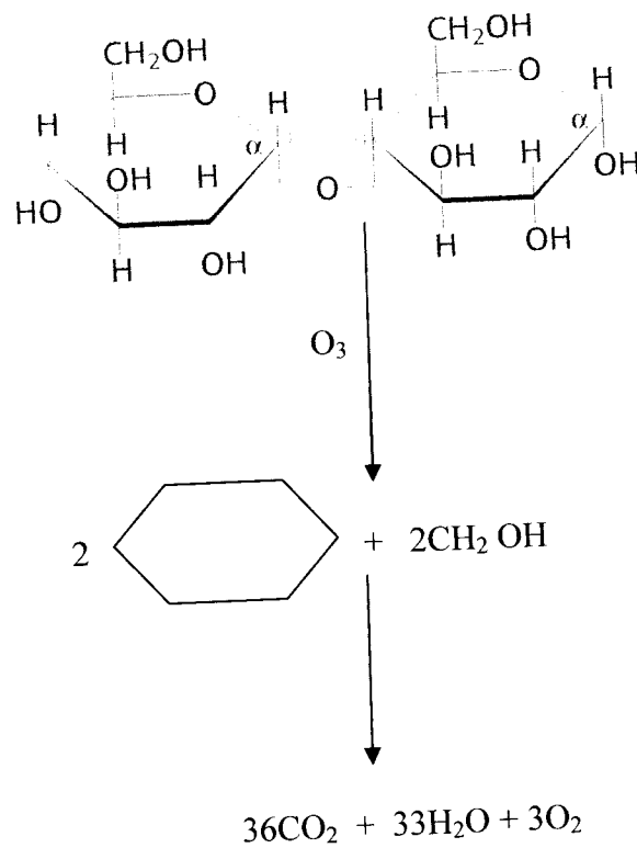
Gambar 4.10. Fenomena Degredasi Maltosa
