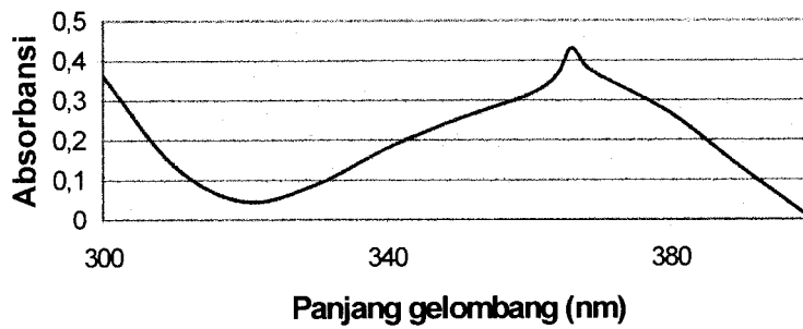
Grafik Spektrum Absorbansi I 2
