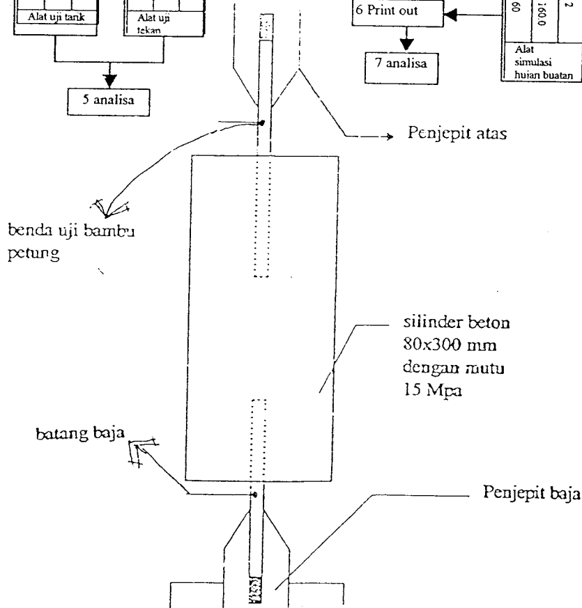
Gambar II.12 contoh penggunaan kayu/bambu sebagai bahan alternatif tulangan beton (sumber: observasi lapangan)
