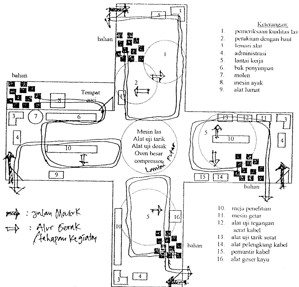
Gambar III.5 Skema penataan peralatan dan sirkulasi pelaku
